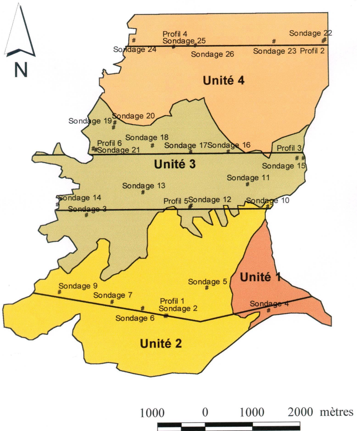
Figure 13 : Carte des unités, transects, sondages et profils.
