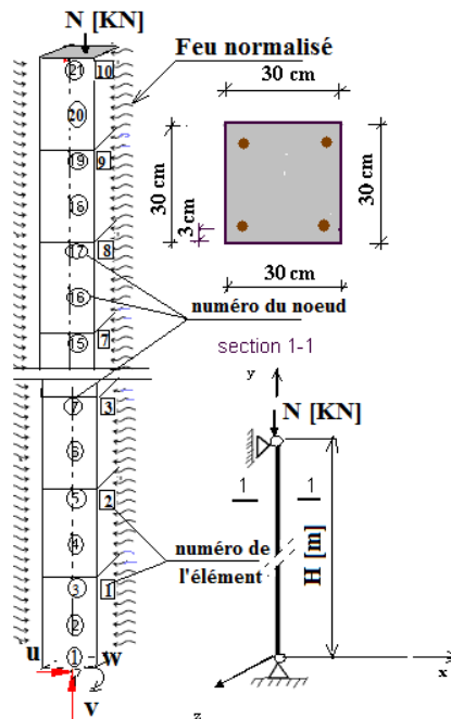
Figure 5. Schématisation des colonnes considérées
