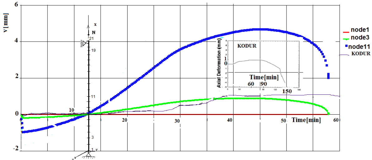
Figure 8. Déplacements verticaux (axiaux) des nœuds 1, 3, 11
