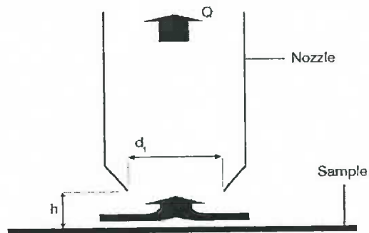
Figure 4. The fluid dynamic gauging — Le jaugage dynamique .
