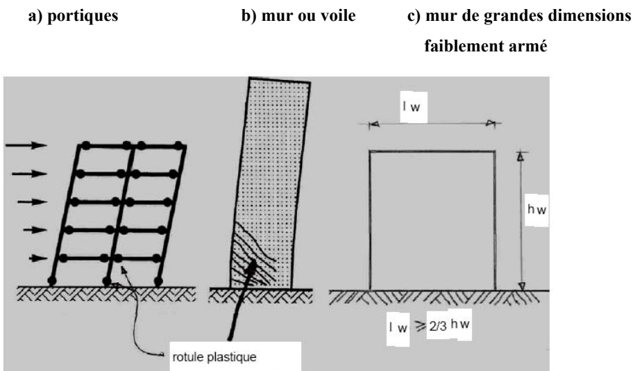
Figure 10.6. Les 3 types fondamentaux de structures parasismiques en béton armé.
