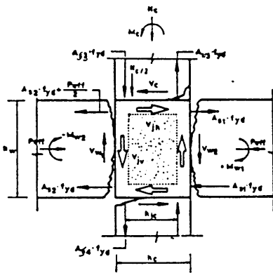
Figure 10.24. Sollicitation de cisaillement du nœud poteau-poutre. Figure 10.25. Etat Limite Ultime d'un nœud correctement armé dans une situation « poutre forte - poteau faible ».
