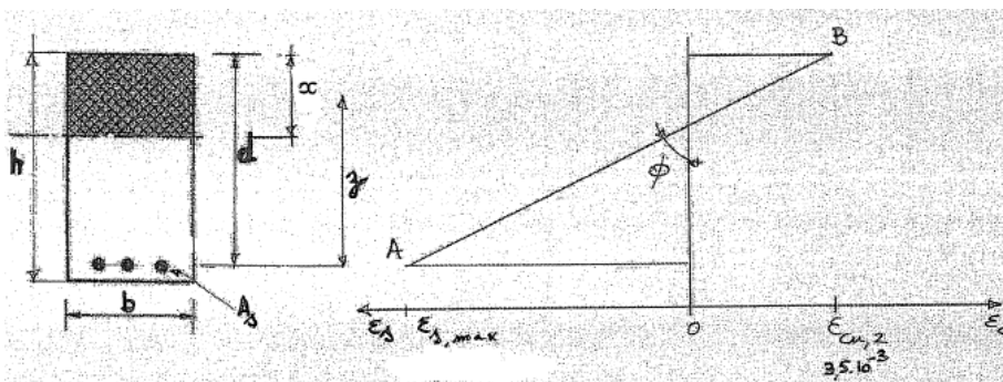
Figure 10.10. Diagramme des \epsilon dans une section fléchie.
