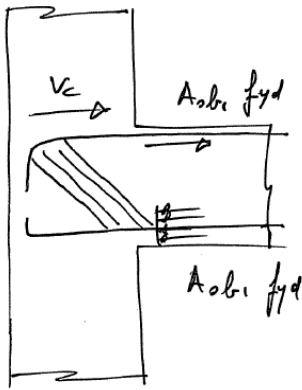
Figure 10.28 d). Mécanismes de transfert d'effort à un nœud de rive.
