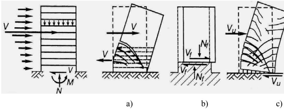
Figure 10.33. Modes de ruine dans les murs ductiles :
