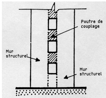
Figure 10.42 . Poutres de couplage.
