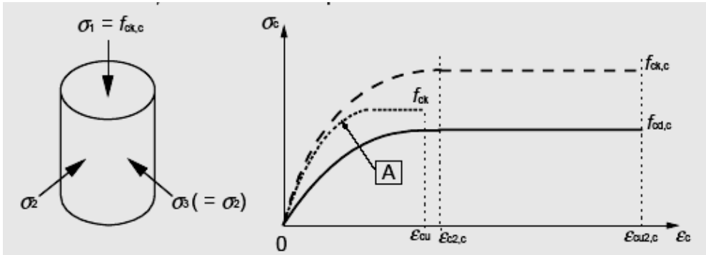
A: f_{ck} , non confiné ; f_{cd} = f_{ck}/1,5
