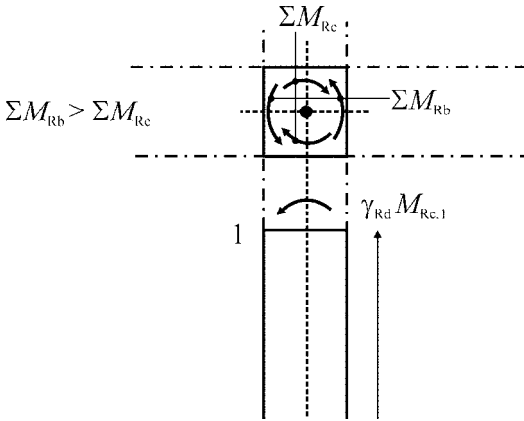
Figure 10.22. Moments M_{i,d} dans la section 1 du poteau pour le calcul de l'effort tranchant sollicitant de calcul du poteau dans le cas « poutres fortes – poteaux faibles ».
