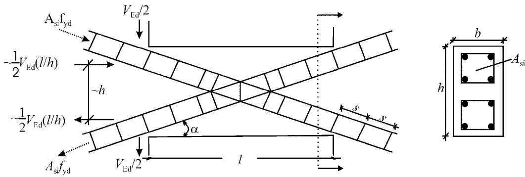
Figure 10.43. Linteau avec armatures diagonales.
