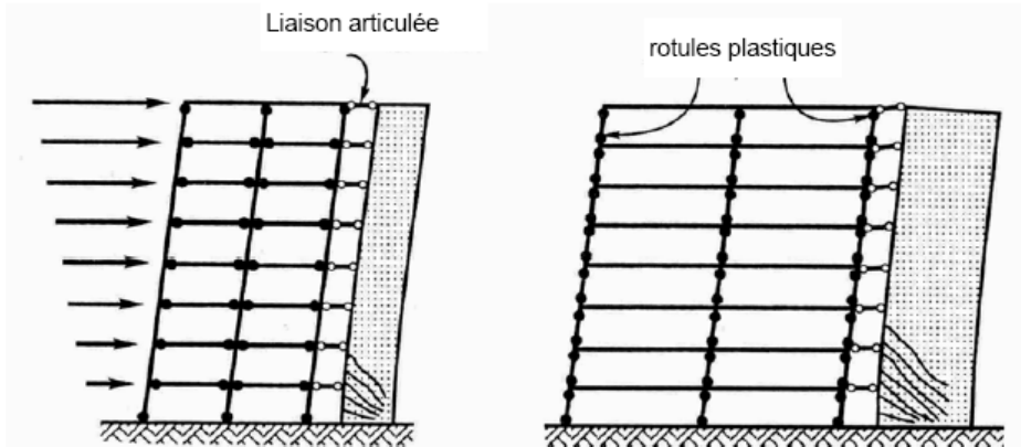
Figure 10.8. Système à contreventement mixte.
