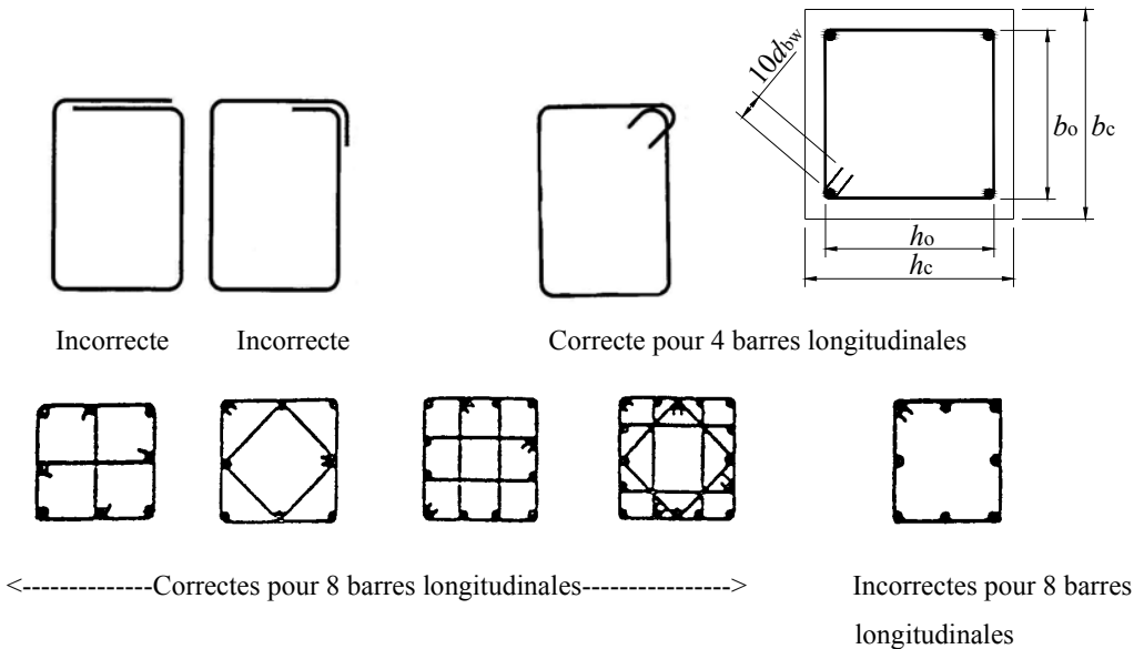
Figure 10.9. Armatures de confinement correctes et incorrectes.
