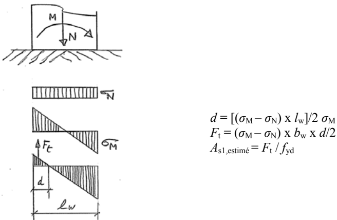
Figure 10.34. Détermination approchée de la résultante de traction en base d'un mur.
