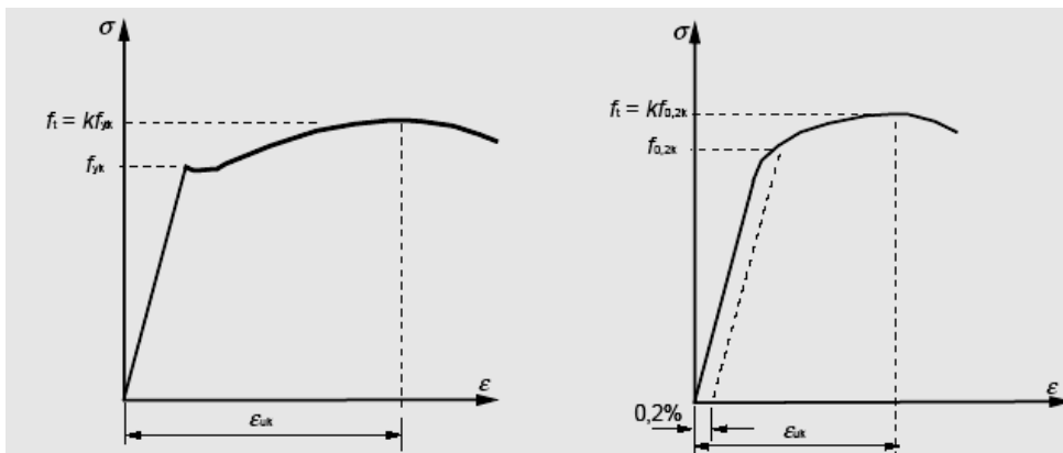
Figure 10.2. Diagrammes contrainte- déformation des aciers à béton.
