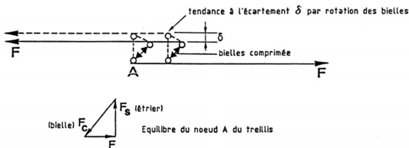
Figure 10.5. Transfert d'effort par recouvrement de barres.
