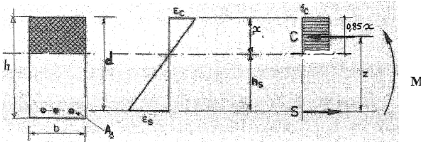
Figure 10.11. Equilibre de la section fléchie.
