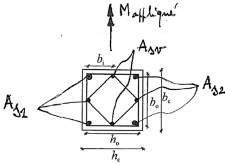
Figure 10.14. Notations pour la section de poteau.
