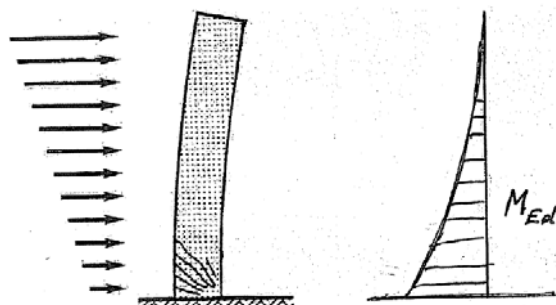
Figure 10.29. Mur ductile et rotule plastique en base.
