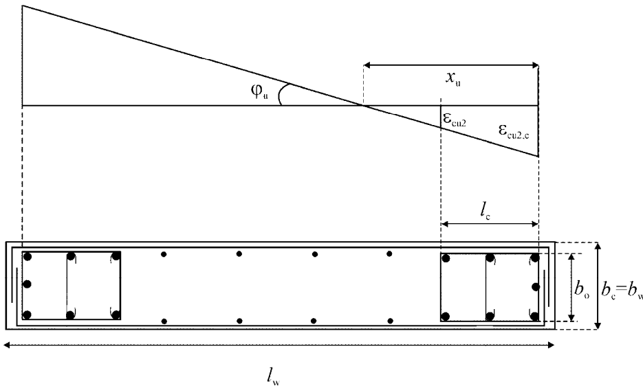
Figure 10.36. Eléments de rive confinés d'une extrémité de mur à bords libres
