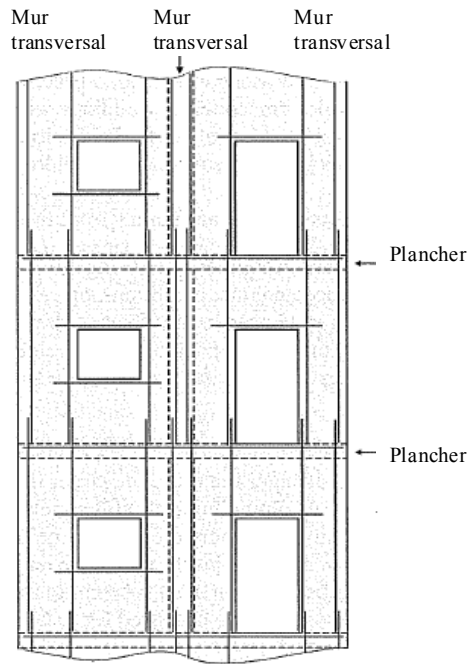
Figure 10.41. Disposition des chaînages
