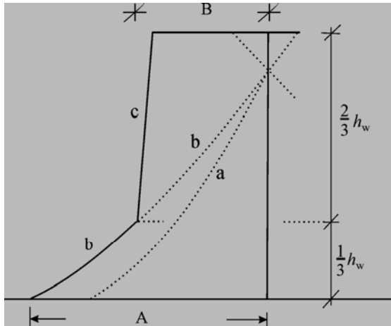
Figure 10.31. Enveloppe de calcul des efforts tranchants dans les murs d'un système à contreventement mixte.
