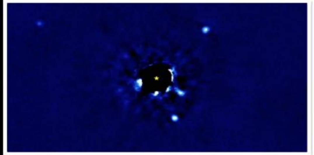
HR 8799
