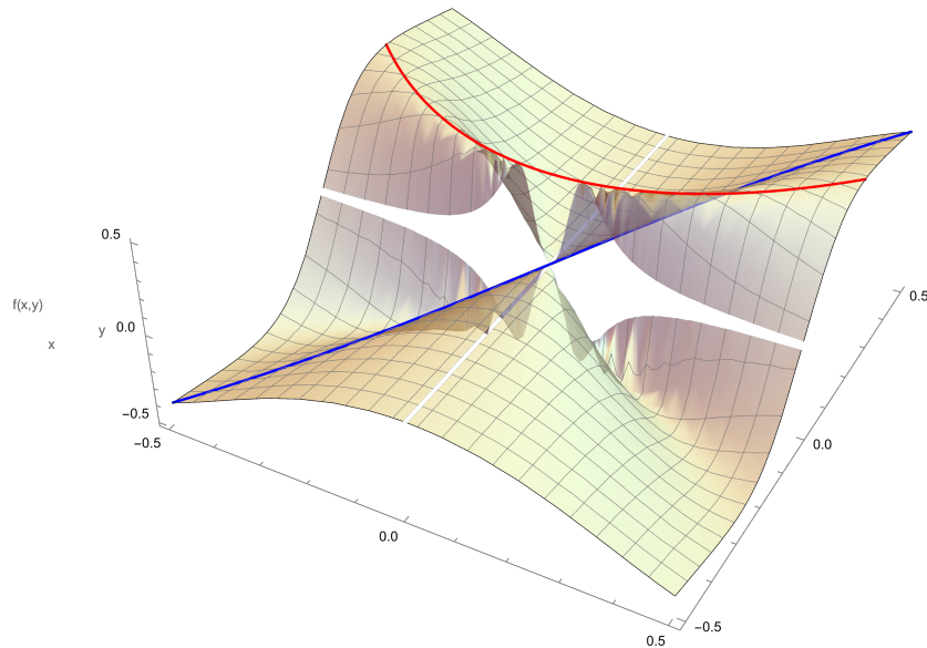
FIGURE 8.2 – Comportement autour de l'origine de la fonction f(x, y) = \frac{x^2y}{x^4+y^2} , montrant deux trajectoires vers (0, 0) : en bleu la droite y = x où la limite est 0, et en rouge la parabole y = x^2 où la limite vaut \frac{1}{2} .
