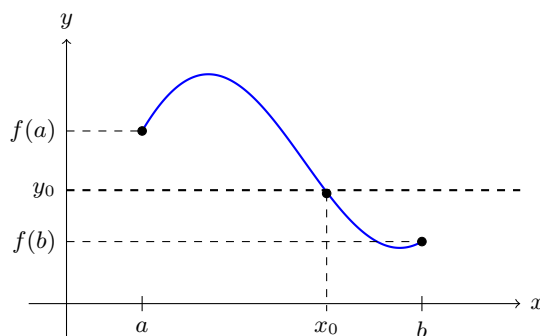
FIGURE 6.4 – Illustration du TVI : Pour y_0 fixé entre f(a) et f(b) , on peut trouver x_0 entre a et b pour lequel f(x_0) = y_0 .
