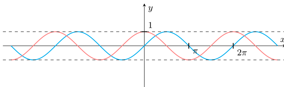
FIGURE 9.6 – Représentation graphique des fonctions sinus (en bleu) et cosinus (en rouge).
