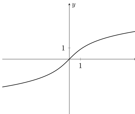
FIGURE 9.16 – Représentation graphique de la fonction arc sinus hyperbolique.
