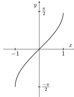
FIGURE 9.10 – Représentation graphique de la fonction arc sinus.
