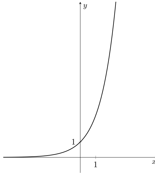
FIGURE 9.1 – Représentation graphique de la fonction \exp réelle.
