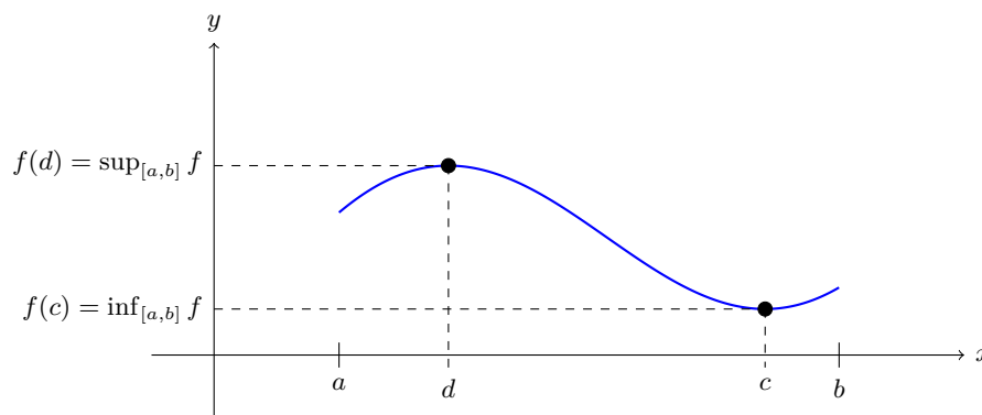
FIGURE 6.3 – Illustration du Théorème des bornes atteintes : la fonction f est bornée sur [a, b] et toutes les valeurs prises par f sur cet intervalle sont comprises entre f(c) et f(d) .
