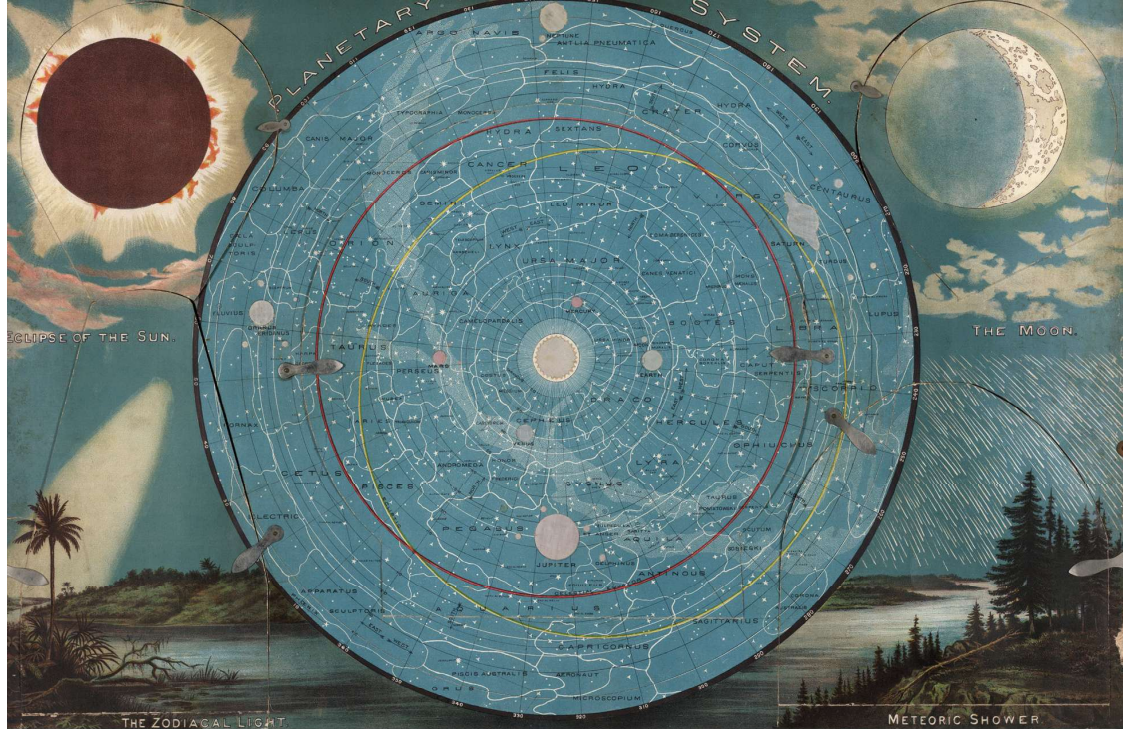
Système planétaire, avec cinq volets à ouvrir, tiré de l'Étude géographique de Levi Walter Yaggy, 1887.
