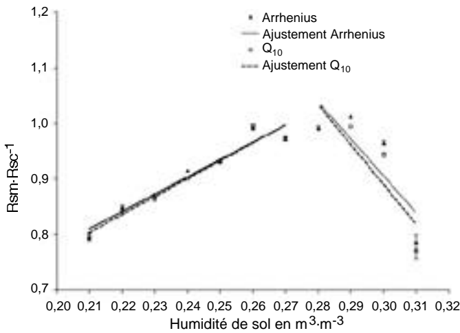
Figure 5. Relation entre les flux de respiration du sol Normalisés par la relation à la température en Q_{10} et la loi d'Arrhénius (rapport des flux mesurés R_{sm} aux flux calculés par le modèle R_{sc} ), et l'humidité de sol en m^3 \cdot m^{-3} . Les données sont agrégées par classes d'humidité avec une résolution de 0,1 m^3 \cdot m^{-3} , sur 22.927 mesures. Les droites représentent les ajustements linéaires — Relationship between soil respiration fluxes, which are standardized with the temperature relationship in Q_{10} and Arrhenius' law (ratio of the R_{sm} measured fluxes to the R_{sc} calculated fluxes), and soil moisture content in m^3 \cdot m^{-3} . The data are aggregated by moisture content classes with a 0.1 m^3 \cdot m^{-3} resolution out of 22,927 measurements. The lines represent linear adjustments.
