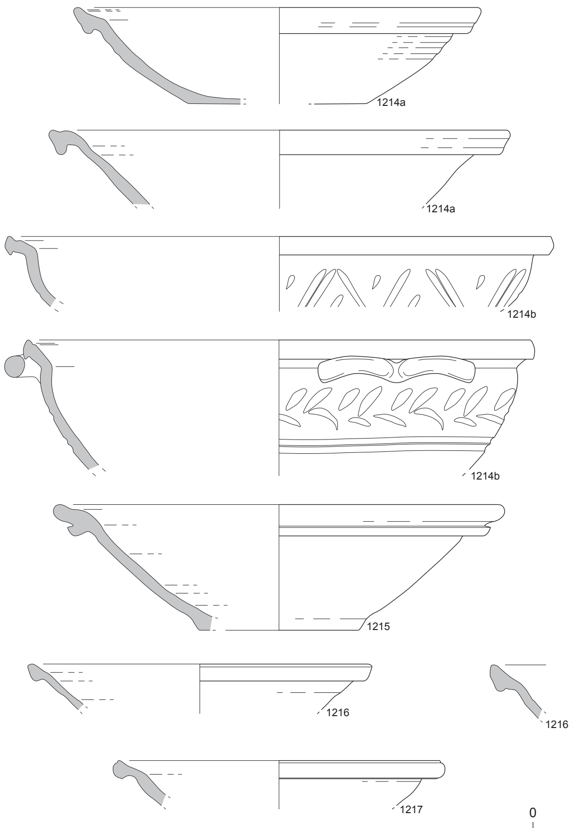
Typologie de la céramique commune claire de la région romaine. Groupe 1200 : bassins et mortiers sans collerette.
