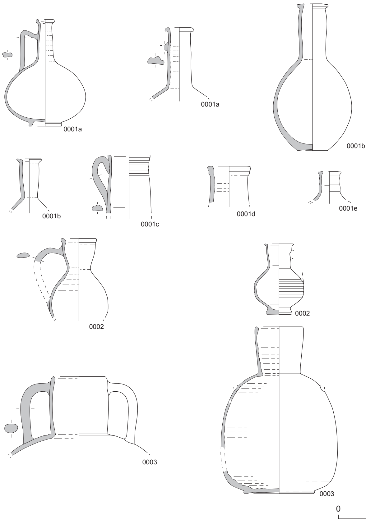
Typologie de la céramique commune claire de la région romaine. Groupe 0000 : cruches non polylobées.
