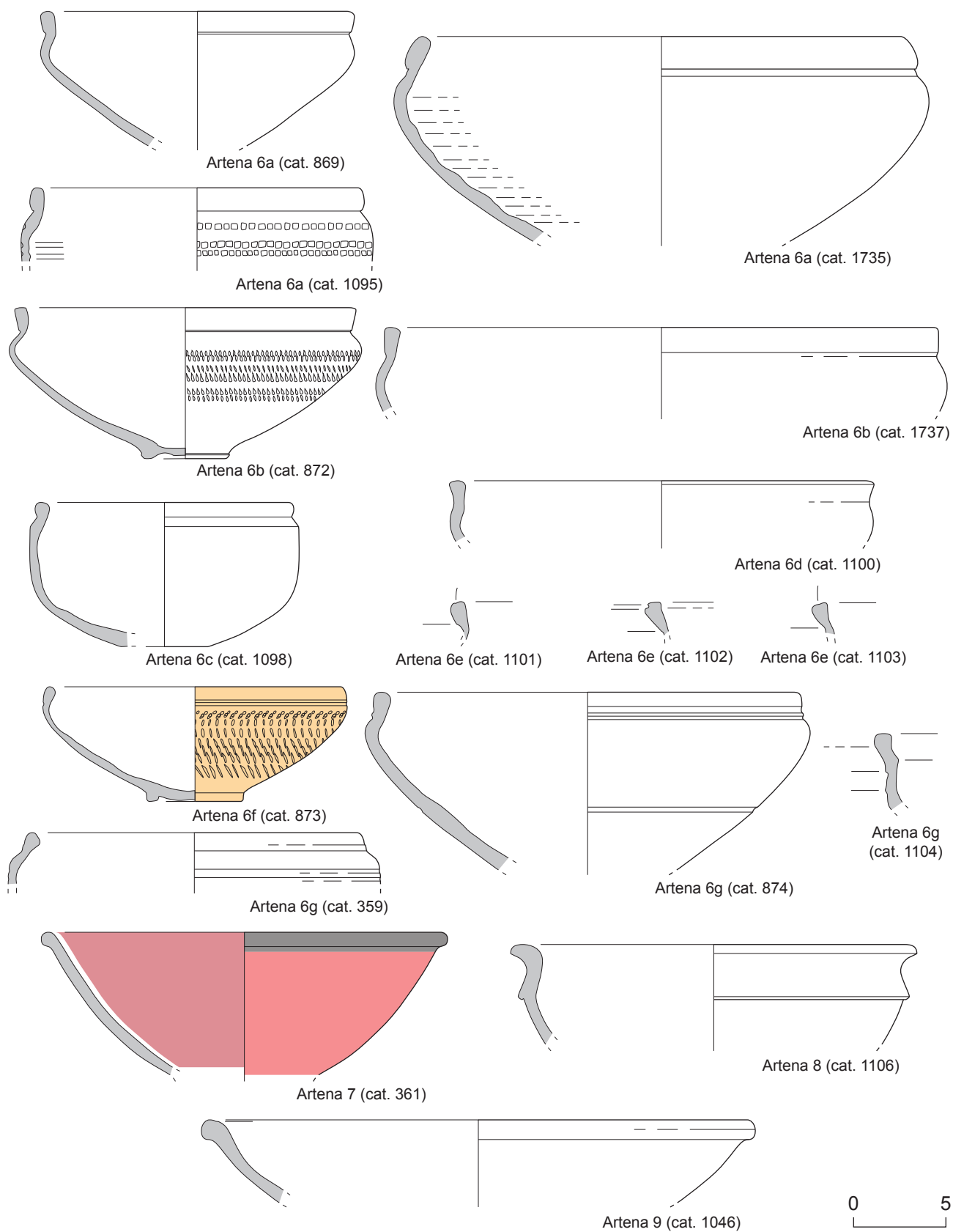
Typologie de la céramique commune claire de la région d'Artana.
