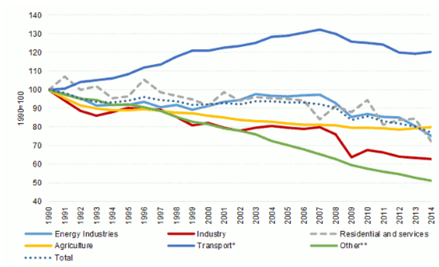
Evolution des émissions CO 2 (Base: 1990, Source: EAA)
