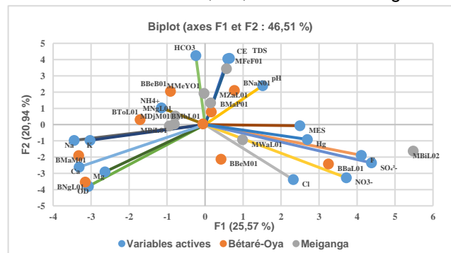
Figure 3 : ACP des variables sur le plan factoriel F1-F2
