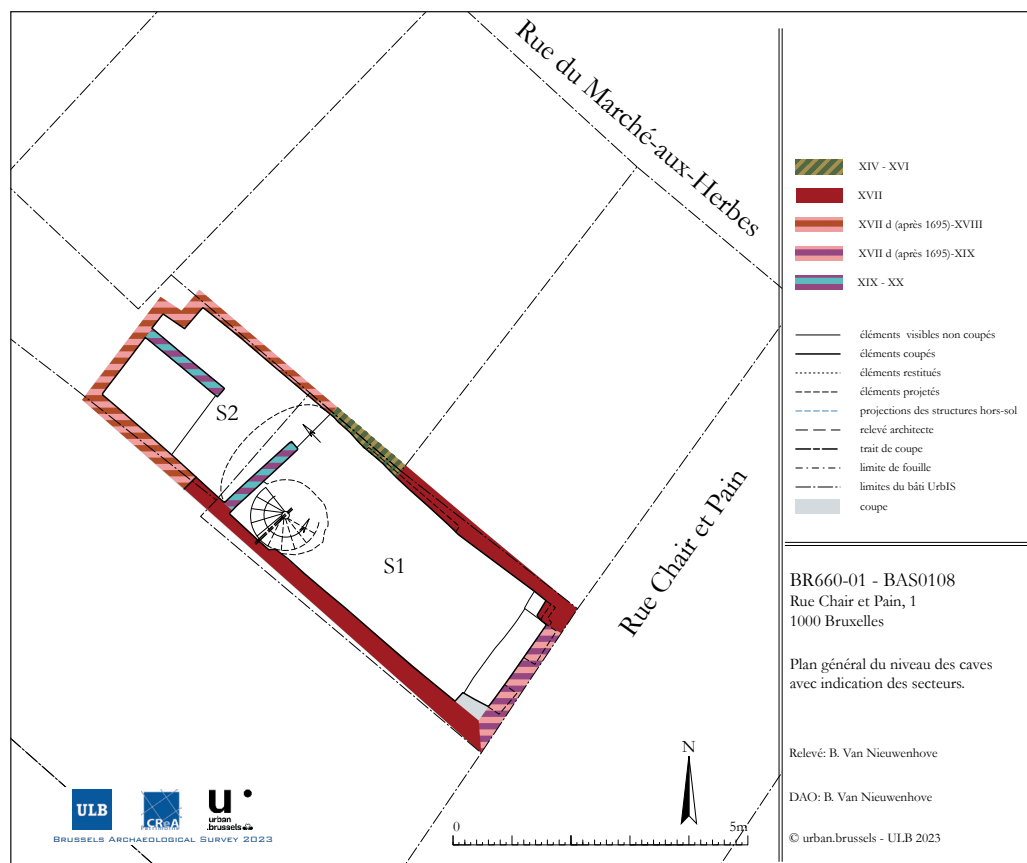
Fig. 71. Plan général des caves avec indication des différentes phases (© urban.brussels-ULB; DAO B. Van Nieuwenhove)
