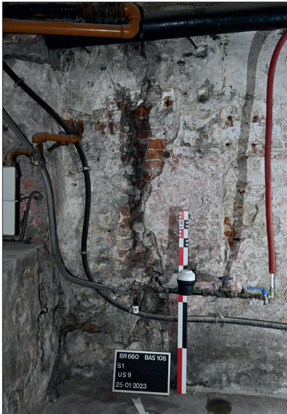
Fig. 10. Vue partielle de la maçonnerie US09, observée au travers d'une saignée (secteur 1) (© urban.brussels-ULB)
