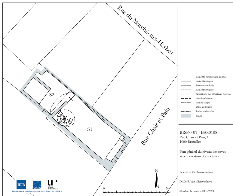
Fig. 5. Plan général des caves avec indication des numéros de secteurs
