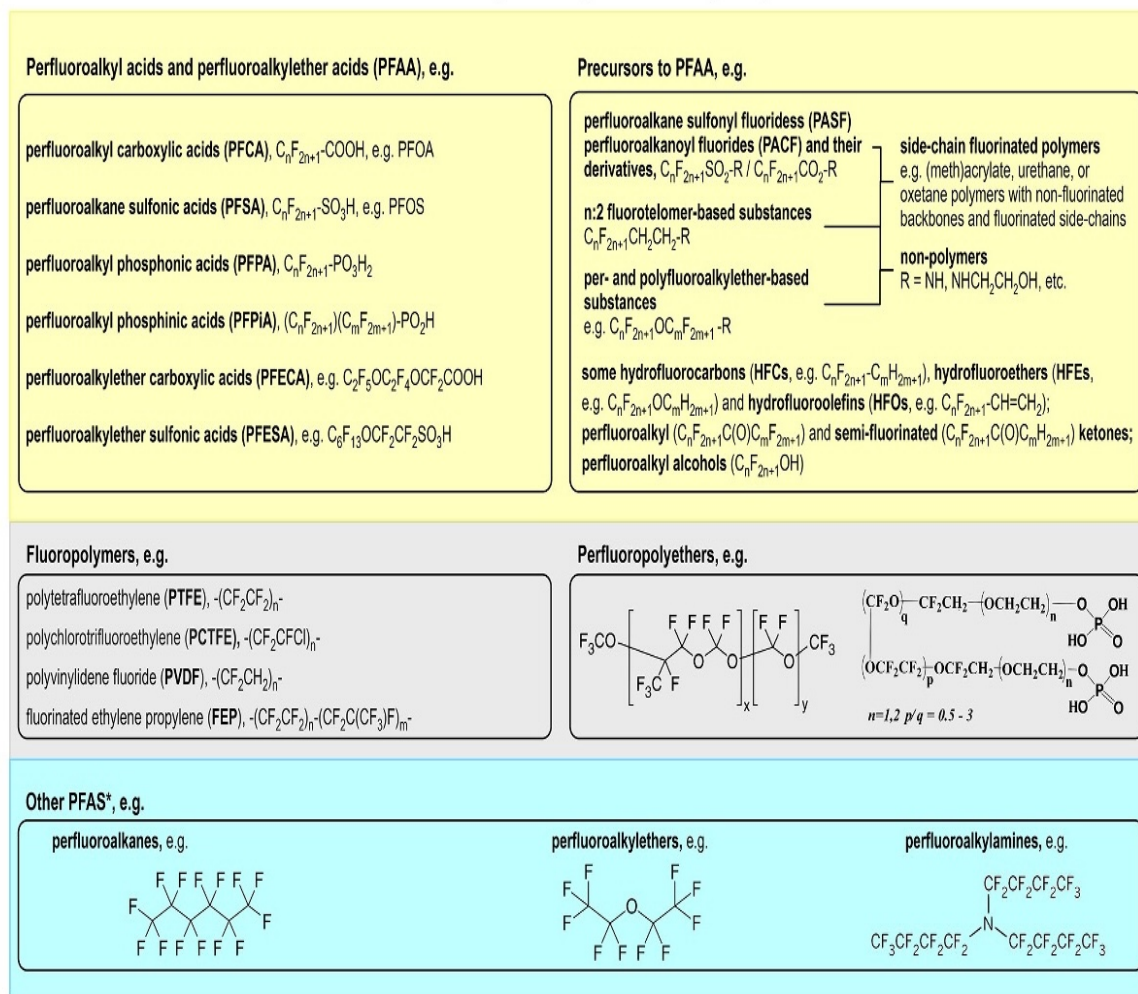
Figure 2. Principales catégories de PFAS et exemples de molécules pour chaque catégorie. Figure reproduite de Environ. Sci. Technol. Lett. 2020, 7, 8, 532-543 ( https://pubs.acs.org/doi/10.1021/acs.estlett.0c00255 ) avec l'aimable autorisation de l'ACS. Avis aux lecteurs souhaitant réexploiter cette image : toute autorisation supplémentaire concernant le matériel extrait doit être adressée à l'ACS.
