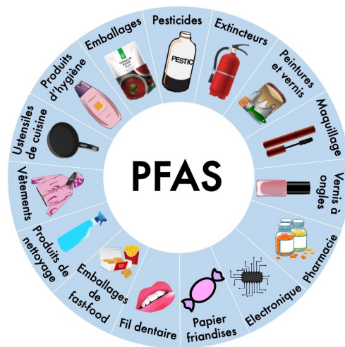
Figure 3. Illustration des principales applications des PFAS. Le document téléchargeable ici reprend les principaux PFAS utilisés, leur structure chimique, et tous les champs applicatifs par catégorie de molécules.
