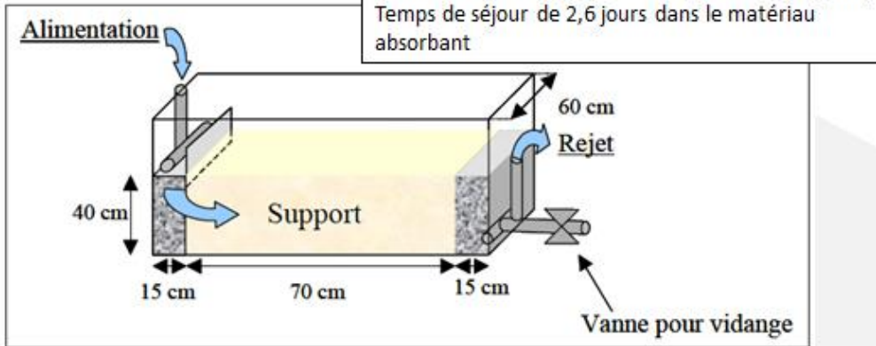
Figure 11 : Dispositif expérimental. (Molle, 2003)
