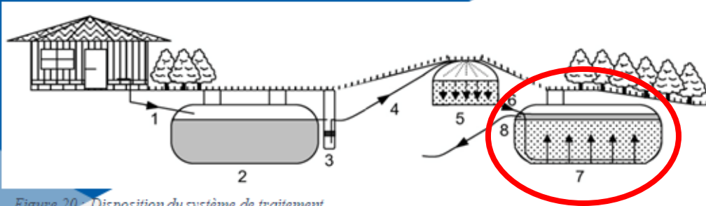
Figure 20 : Disposition du système de traitement.
