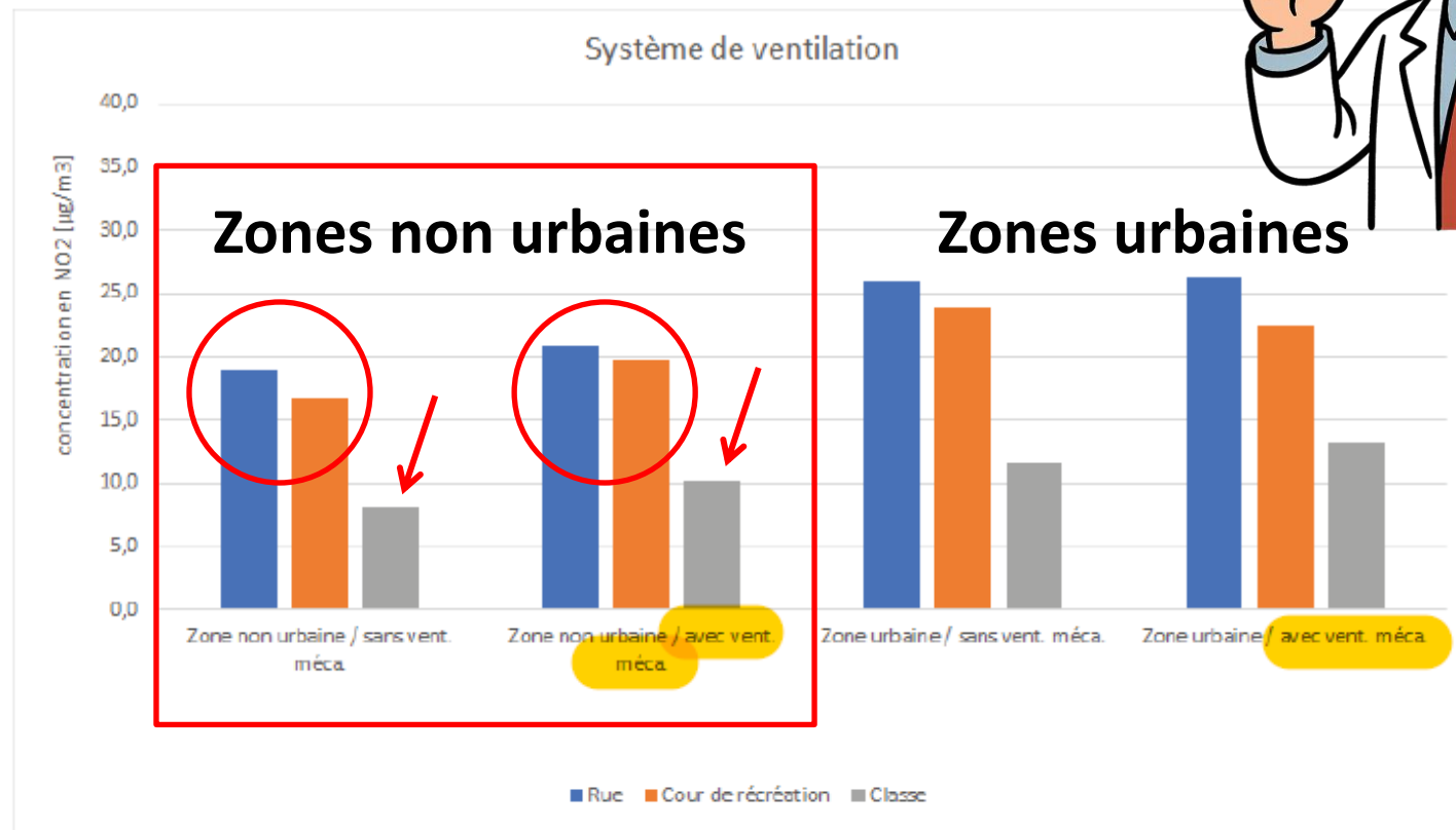
Figure 6.3 Comparaison des concentrations moyennes en NO 2 dans les zones urbaines et non urbaines, avec ou sans système de ventilation mécanique.
