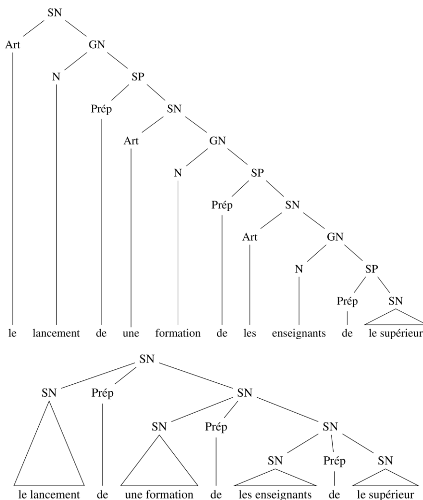
Figure 9. – Arbres ACI comportant des compléments déterminatifs récursifs (premièrement, selon la règle SP \rightarrow \text{Prép SN} ; deuxièmement, selon la règle SN \rightarrow \text{SN Prép SN} ).
