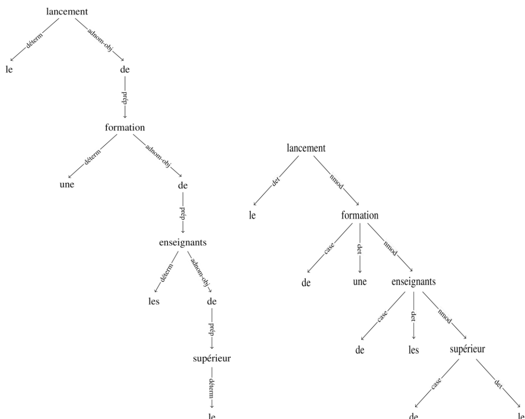
Figure 10. – Arbres dépendanciels comportant des compléments déterminatifs récursifs (premièrement, selon la Théorie Sens-Texte ; deuxièmement, selon les Universal Dependencies ).
