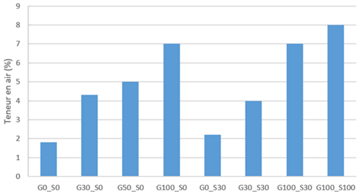
Figure 4.2 Teneur en air des bétons avec MIOM
