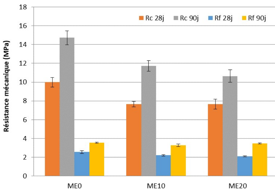
Figure 2.3 Résistance mécanique des mortiers d'enduit avec CEM II 32,5 et cendres volantes de biomasse
