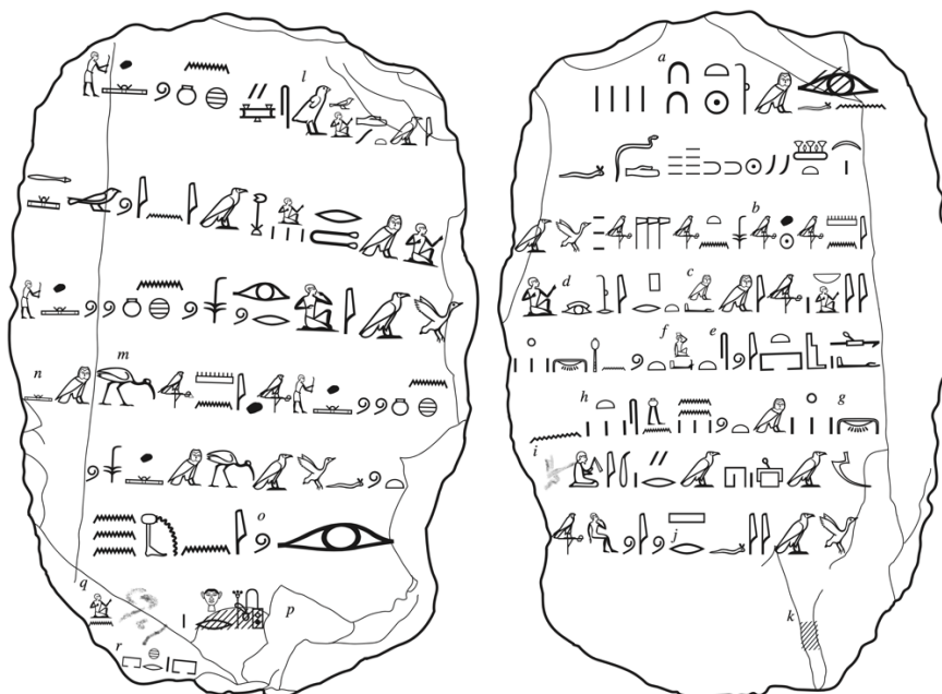
Fig. 3. Transcription hiéroglyphique de l'O. VoK 2022.13 r° et v°
