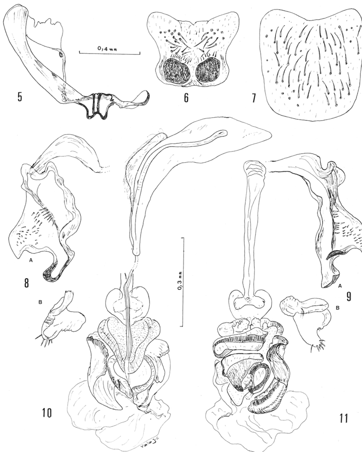
Fig. 5 à 11 Euthycera flavostriata . 5 épandrium. 6 cinquième sternite. 7 quatrième sternite. 8 processus de l'hypandrium en vue postérieure : 8 a processus antérieur, 8 b processus postérieur. 9 idem en vue antérieure : 9 a processus antérieur, 9 b processus postérieur. 10 édéage en vue postérieure, 11. édéage en vue antérieure.
