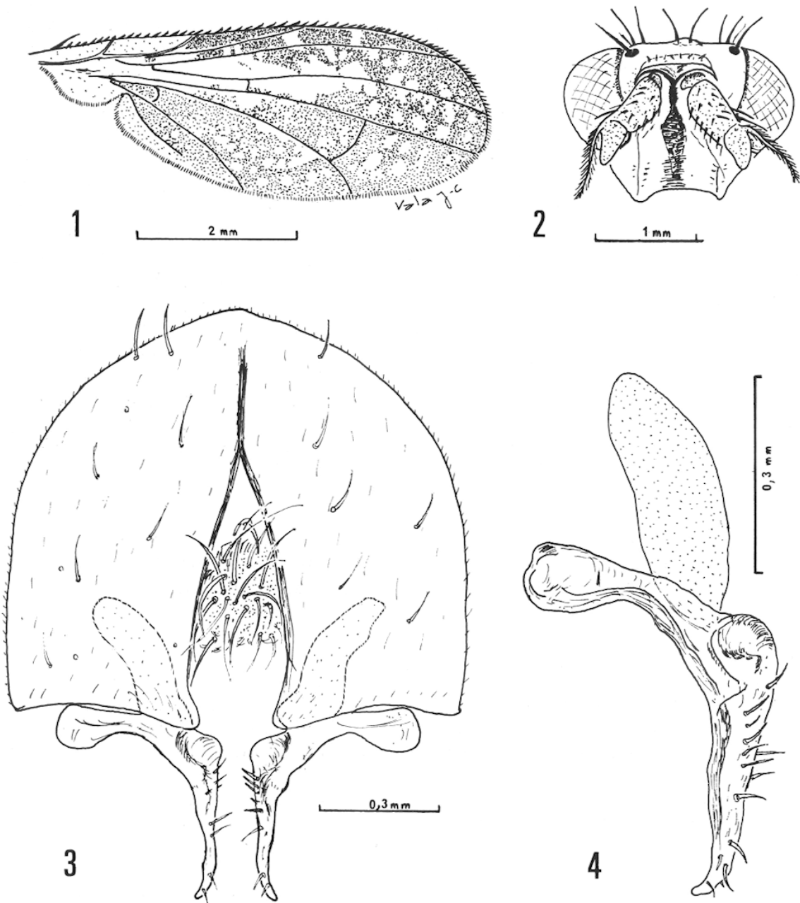
Fig. 1 à 4: Euthycera flavostriata . 1 aile. 2 face. 3 épandrium. 4 forceps externes = surstili.
