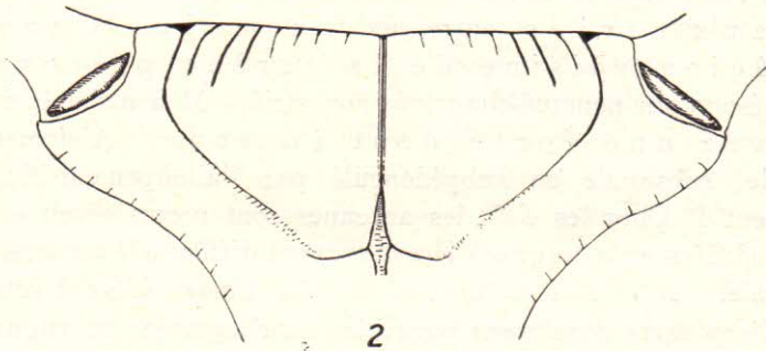
FIG. 1-2. — Partie dorsale du segment médiaire chez deux Ectemnius ( Policrabro ) : 1. forestus n. sp. ♀ ; 2. krusemani (LECLERCQ). (±30 fois.)
