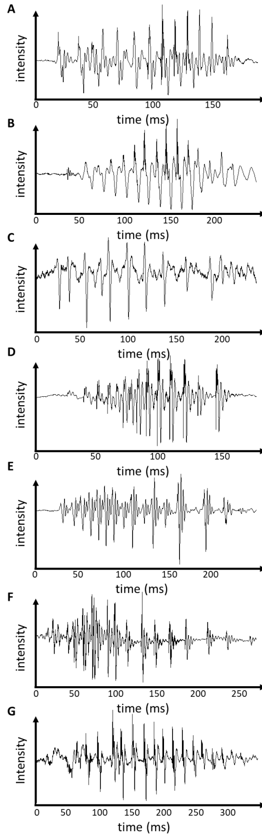
Fig. SP3 Oscillograms of a sound produced by (A) Hypostomus alatus , (B) H. denticulatus , (C) H. francisci , (D) H. margaritifer , (E) H. regani , (F) H. strigaticeps and (G) H. velhochico .
