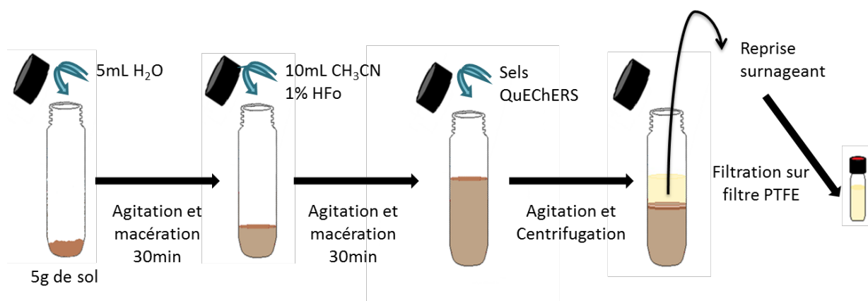
Figure 37. Schéma d'extraction des PPP dans un sol.
