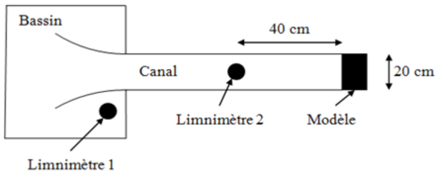
Figure 4. Schéma de la zone d'essai et positionnement des appareils de mesure
