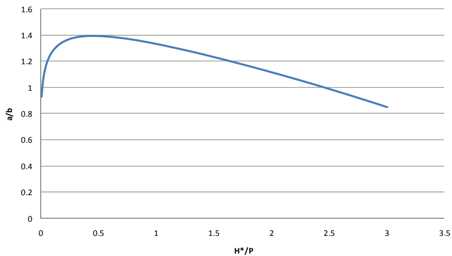
Figure 8. Rapport de forme a/b pour une utilisation optimale du PKW étudié en fonction de la charge adimensionnelle en amont
