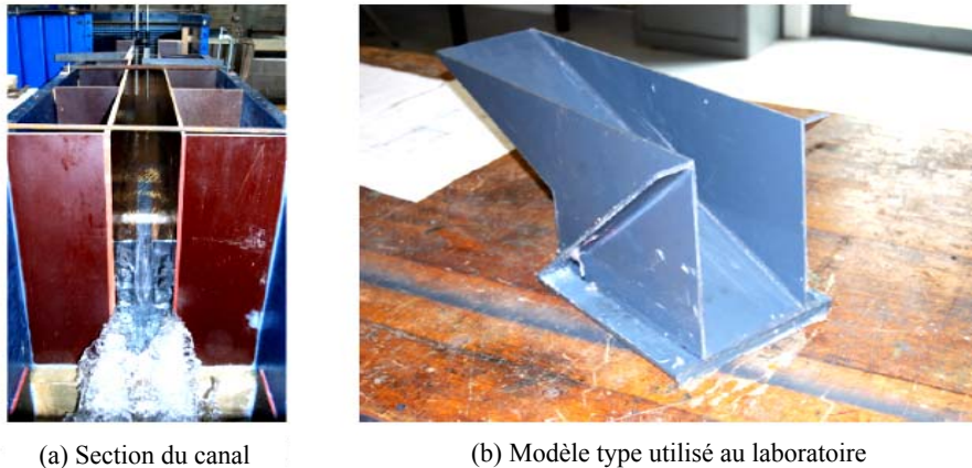
Figure 3. Exemple de modèles étudiés au laboratoire
