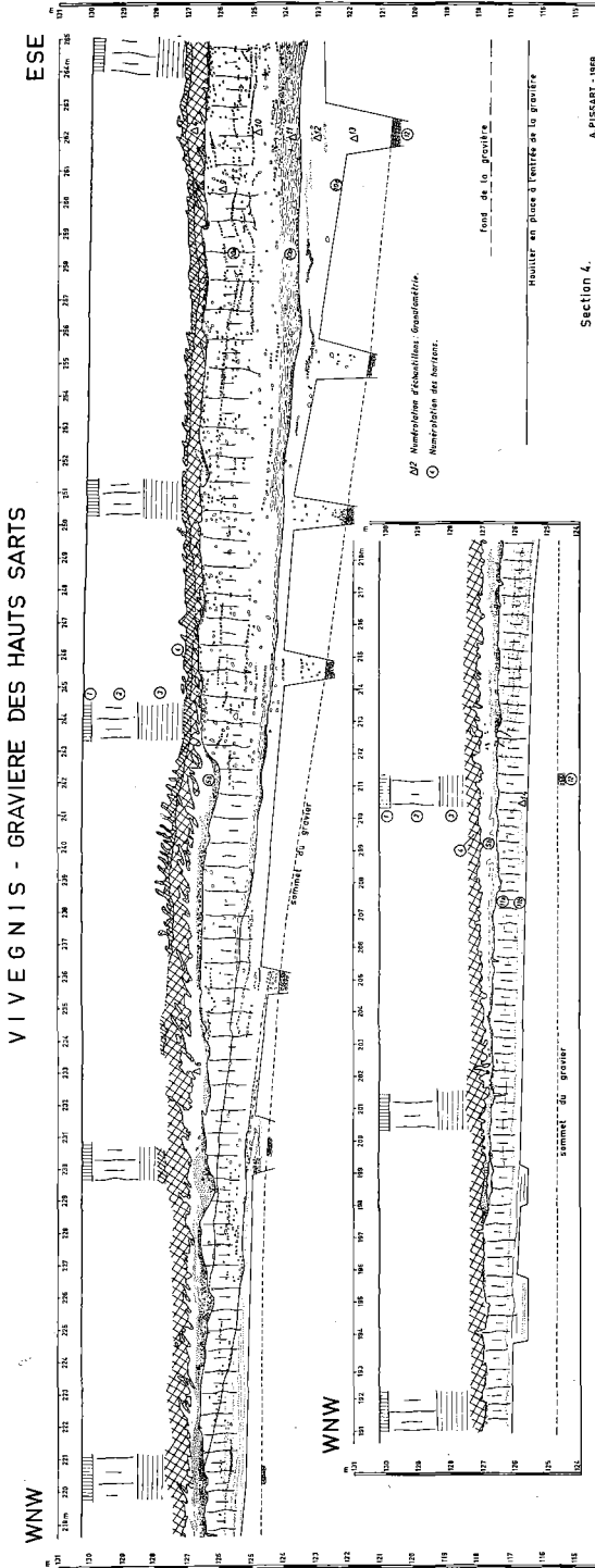
Fig. 5. — Section 4. La localisation de la coupe est donnée sur la figure 1.
