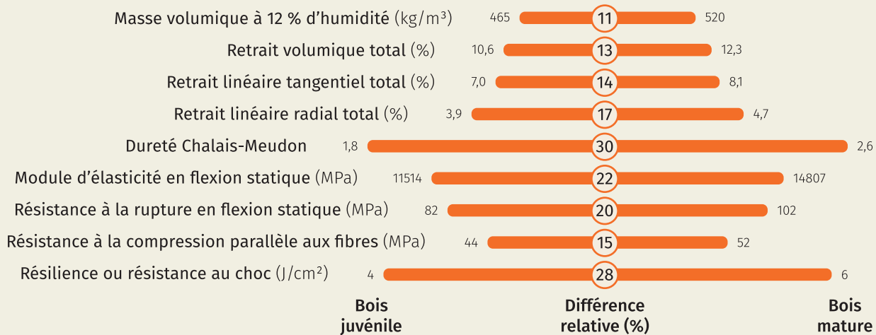
Figure 3. Valeurs moyennes des propriétés physiques et mécaniques de bois de douglas récolté en Wallonie évaluées sur éprouvettes standardisées, en distinguant le bois mature et le bois juvénile (respectivement environ 885 et 275 échantillons).
