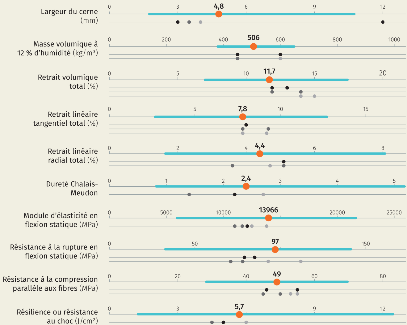
Figure 2. Propriétés physiques et mécaniques du bois de douglas produit en Wallonie, évaluées sur des éprouvettes standardisées sans défauts (nombre d'éprouvettes testées pour chaque propriété : environ 1250).
