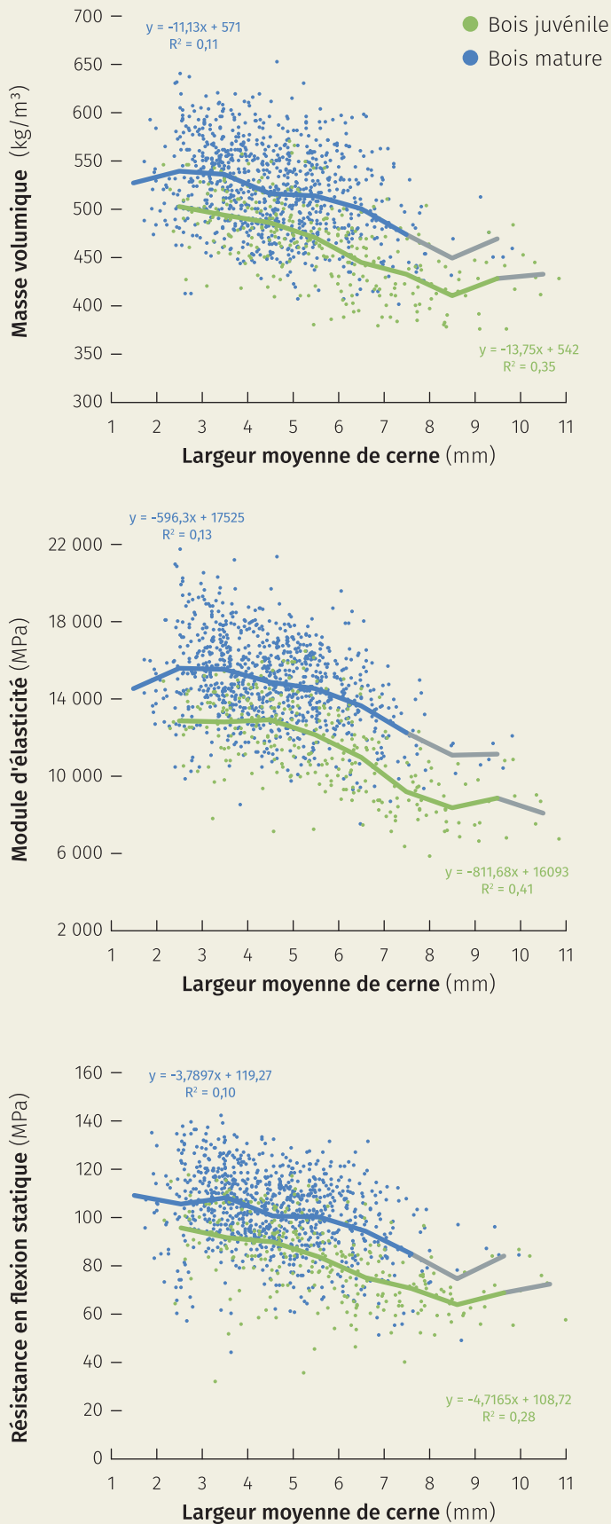
Figures 6, 7 et 8. Influence de la largeur moyenne des cerne sur la masse volumique, le module d'élasticité et la résistance en flexion, dans le bois juvénile (points verts) et le bois mature (points bleus). Les valeurs moyennes par classe de largeur moyenne de cerne sont représentées par les lignes (les valeurs des classes présentant moins de dix observations apparaissent en gris).
