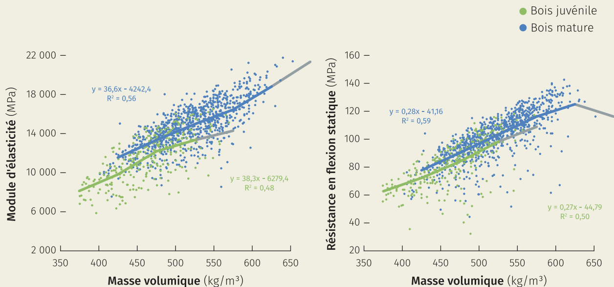
Figures 4 et 5. Influence de la masse volumique sur le module d'élasticité et la résistance en flexion, pour le bois juvénile (points verts) et le bois mature (points bleus). Les valeurs moyennes par classe de masse volumique sont représentées par les lignes (les valeurs des classes présentant moins de dix observations apparaissent en gris).
