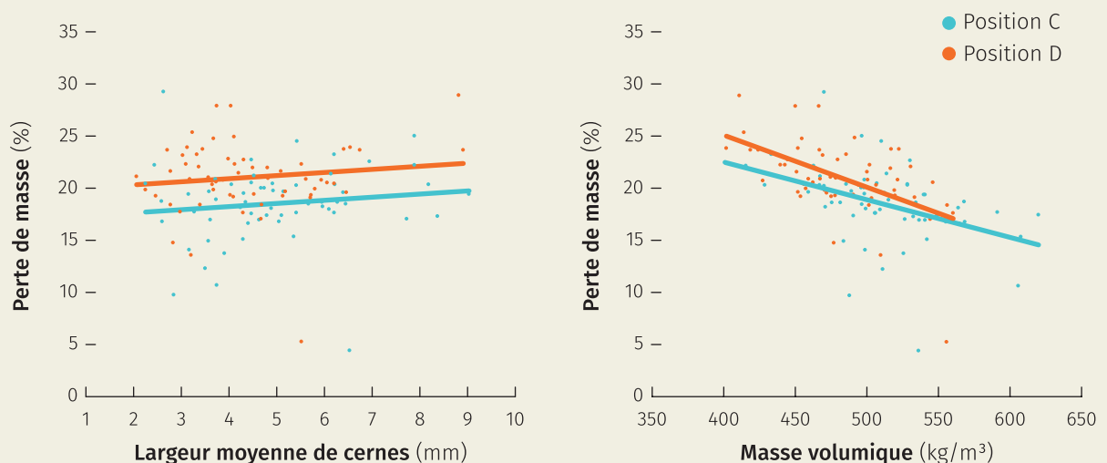
Figure 10. Pertes de masse (%) observées sur les 60 arbres dans les positions C et D, en fonction de la largeur moyenne de cerne (à gauche) et de la masse volumique (à droite).
