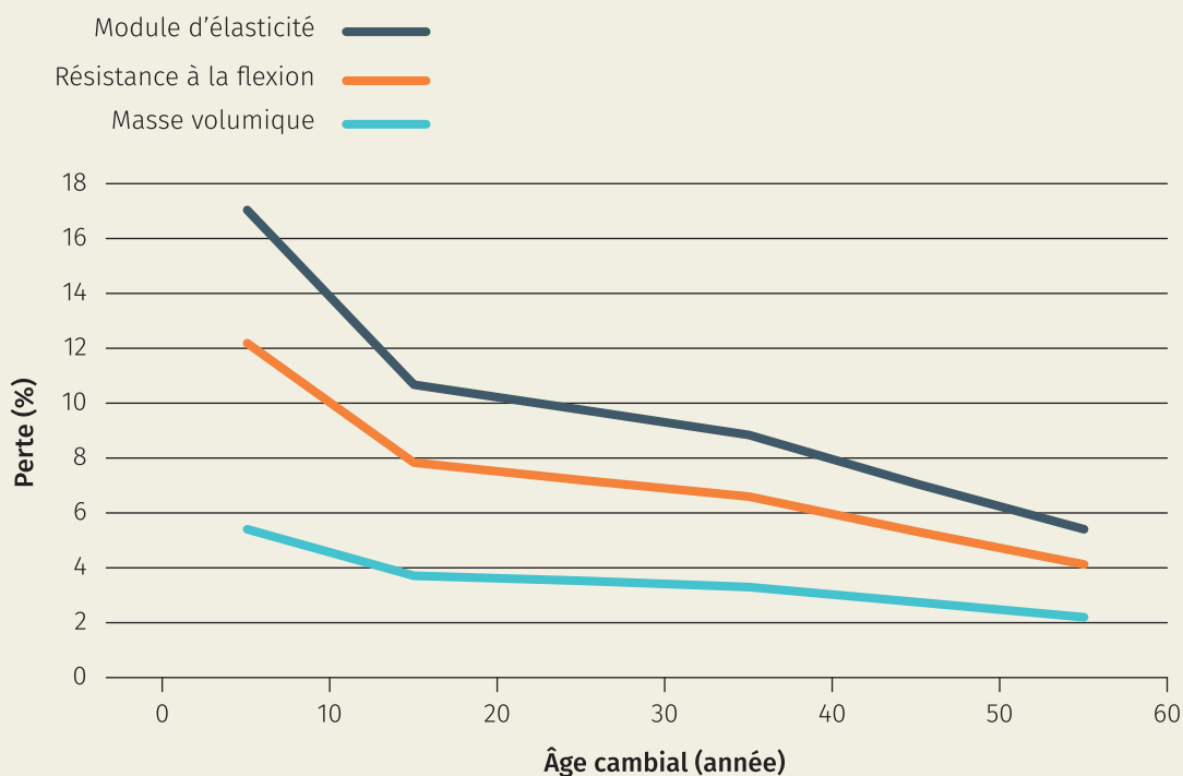
Figure 9. Profil radial de diminution des propriétés physico-mécaniques lorsque l'on compare une vitesse de croissance élevée (25 % supérieure à la moyenne observée dans cette classe d'âge) à une vitesse de croissance faible (25 % inférieure à la moyenne observée dans cette classe d'âge).
