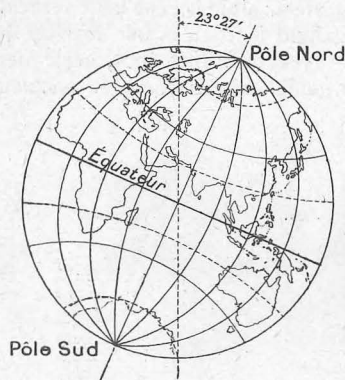
Fig. 3. — Helling der Aardas.
