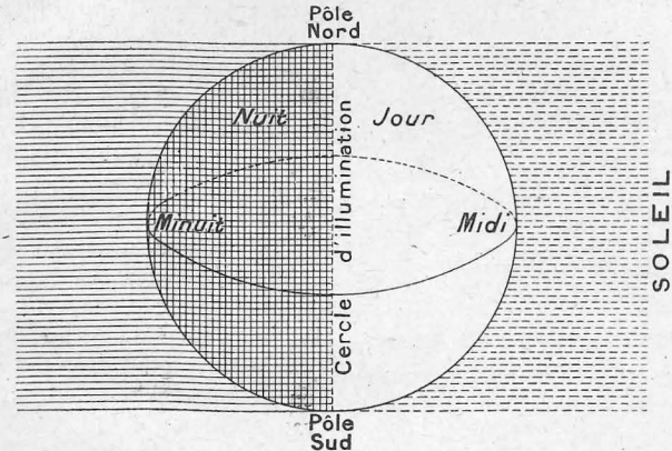
Fig. 2. — Dag en Nacht, op 21 Maart en op 23 September.
