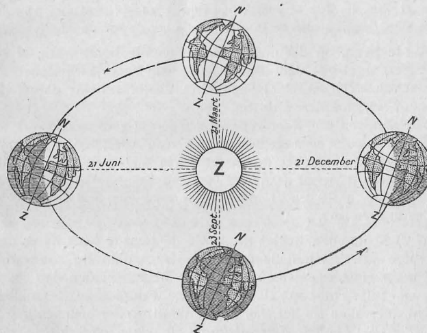
Fig. 5. — De jaargetijden; het parallelisme der aardas.
