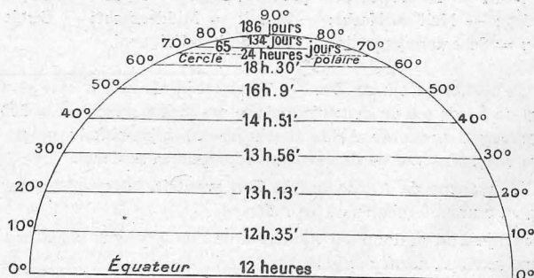
Fig. 4. — Maxima-lengte der dagen in 't Noordelijk halfond.
