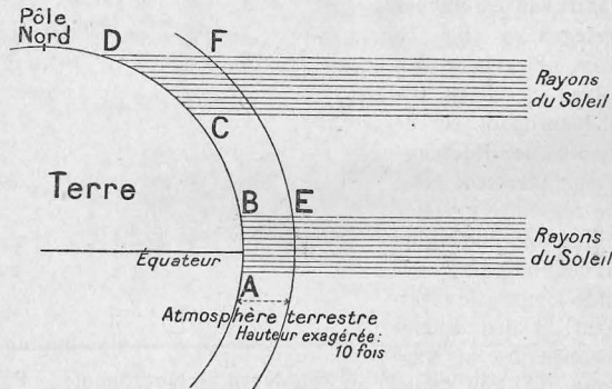
Fig. 8. — Invloed der warmtegraden der Zon op verschillende breedte.
