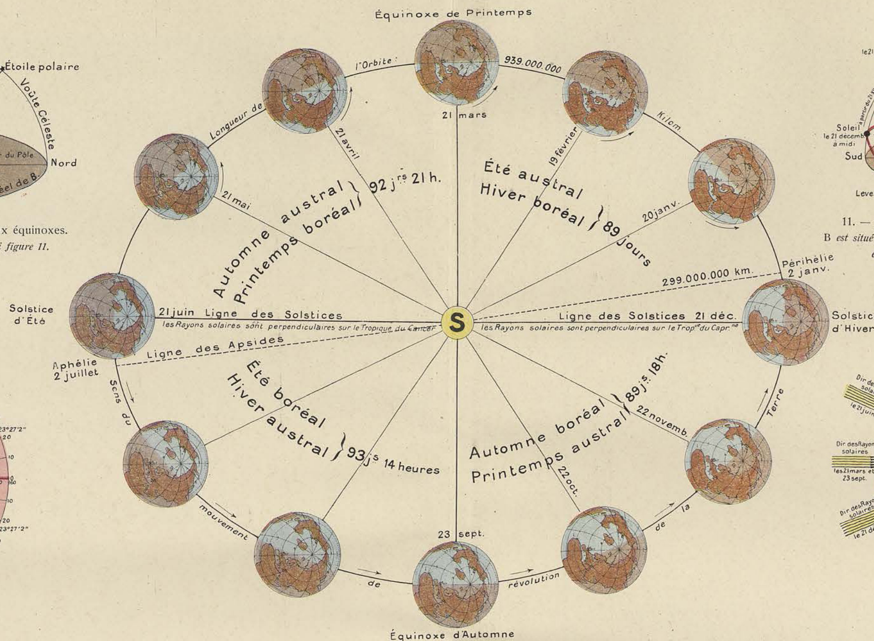
12. — Mouvement de révolution de la Terre autour du Soleil. — Les Saisons. Le point de vue est situé au pôle Nord de l'écliptique, mais l'aplatissement de l'ellipse que parcourt la Terre est exagéré environ 300 fois.
