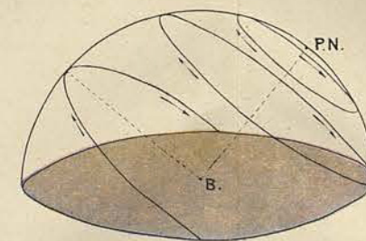
7. — Mouvement apparent d'étoiles vu du 51° lat. N.
