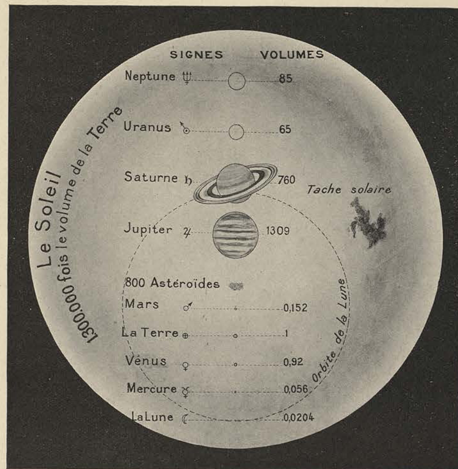
1. — Dimensions comparées du Soleil, des Planètes, de la Lune et de l'orbite lunaire.
