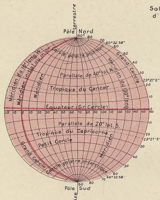
13. — Lignes et Cercles de la Sphère.
