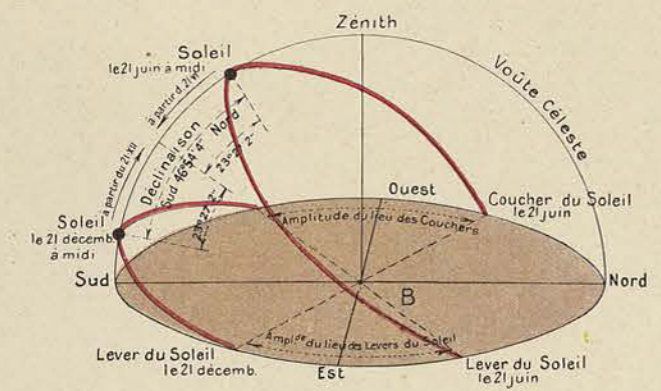
11. — Mouvement apparent du Soleil aux solstices. B est situé par 50° latitude N.; la distance maximum entre l'Est et le lieu du lever du Soleil est de 38° 30'.
