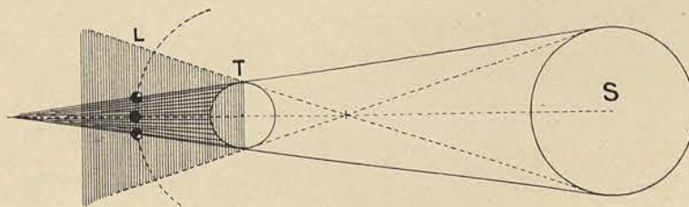
d) Éclipse totale et partielle de la Lune
