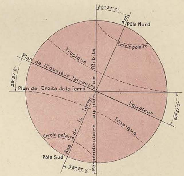
16. — Inclinaison de l'axe de la Terre sur le plan de l'orbite terrestre.
