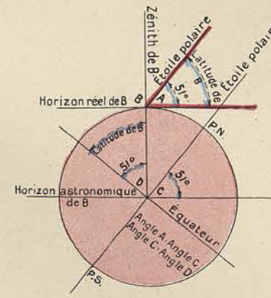
18bis. — La latitude d'un lieu est la hauteur du pôle.
