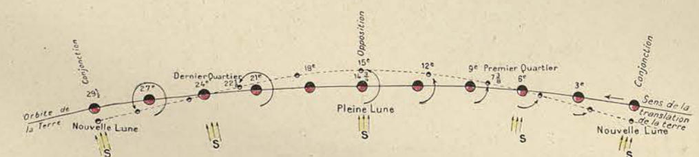
6. — Courbe décrite par la Lune, en un mois lunaire, autour de la Terre.
