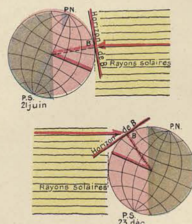
18. — Conséquences de l'obliquité de l'axe terrestre. B est situé par 33° de latitude N.
