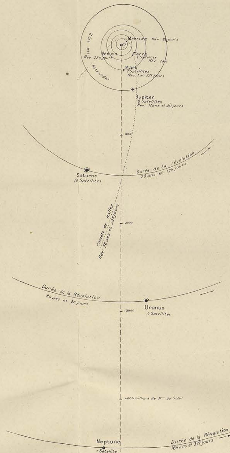
3. — Système solaire ou planétaire.
