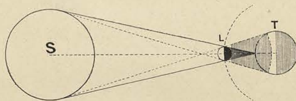
c) Éclipse totale du Soleil pour un seul point de la Terre
