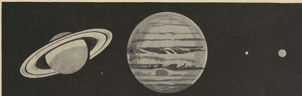
8. Saturne. Jupiter. Mars. Vénus.
