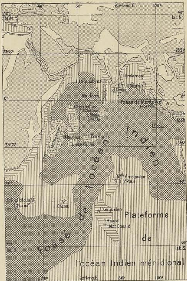
37. — Profondeur des océans (océan Indien)
