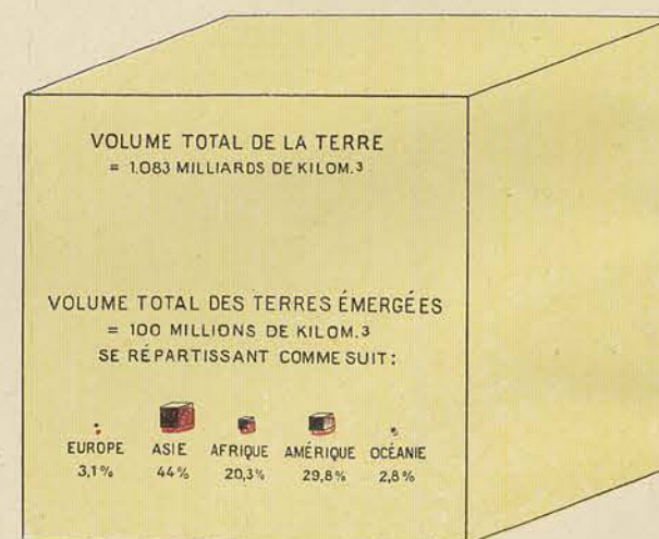
Volumes comparés du Globe et des terres émergées.
