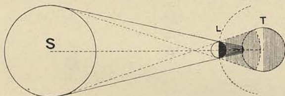
b) Éclipse totale du Soleil pour une région de la Terre et partielle pour d'autres
