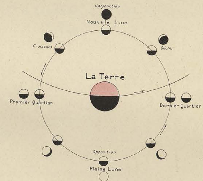
5. — Phases de la Lune.
