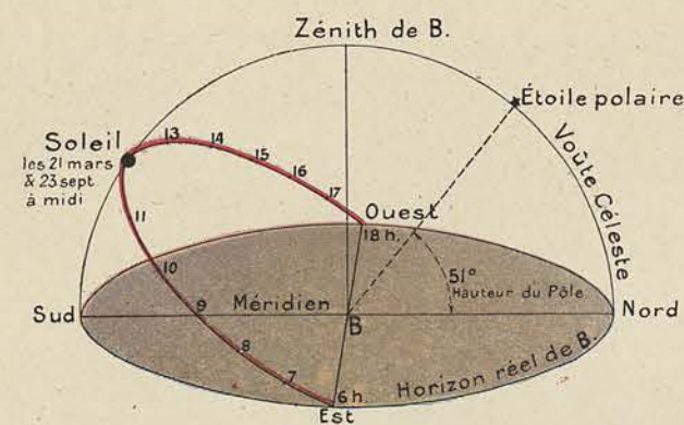
10. — Mouvement apparent du Soleil aux équinoxes. B est situé par 51° latitude N.; voir aussi figure 11.
