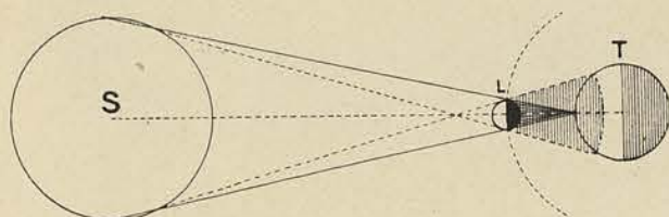
a) Éclipse annulaire du Soleil
