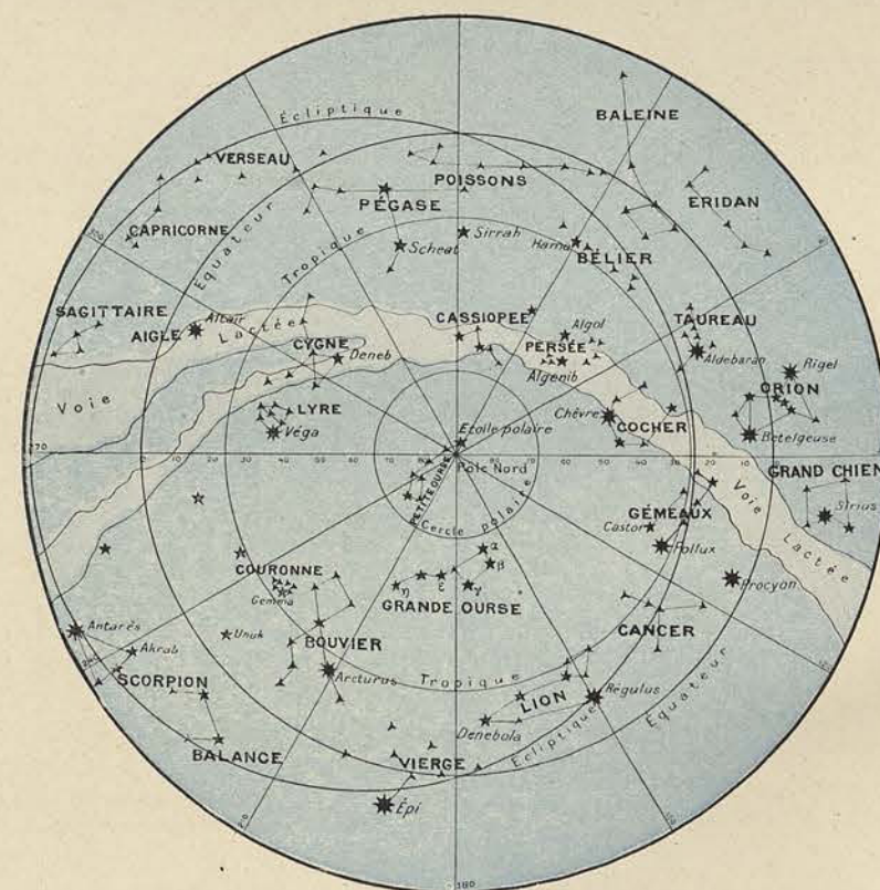
2. — Hémisphère céleste boréal.
