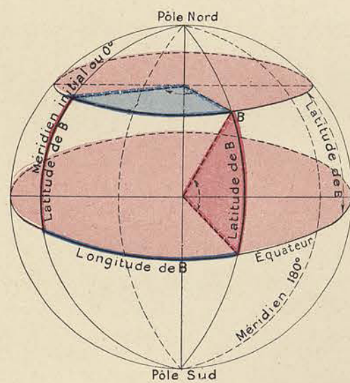
14. — Coordonnées géographiques. Latitude et Longitude.
