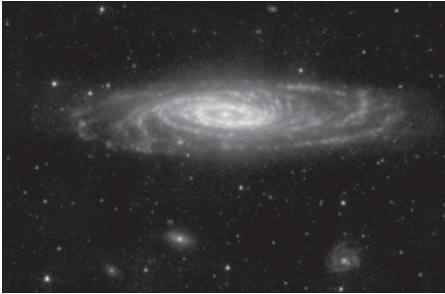
La galaxie NGC7331 en infrarouge (NASA/Spitzer)
