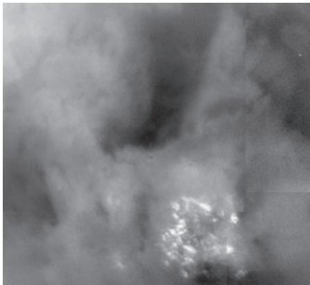
Nuages de méthane
