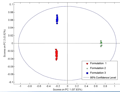
Score plot PCA
