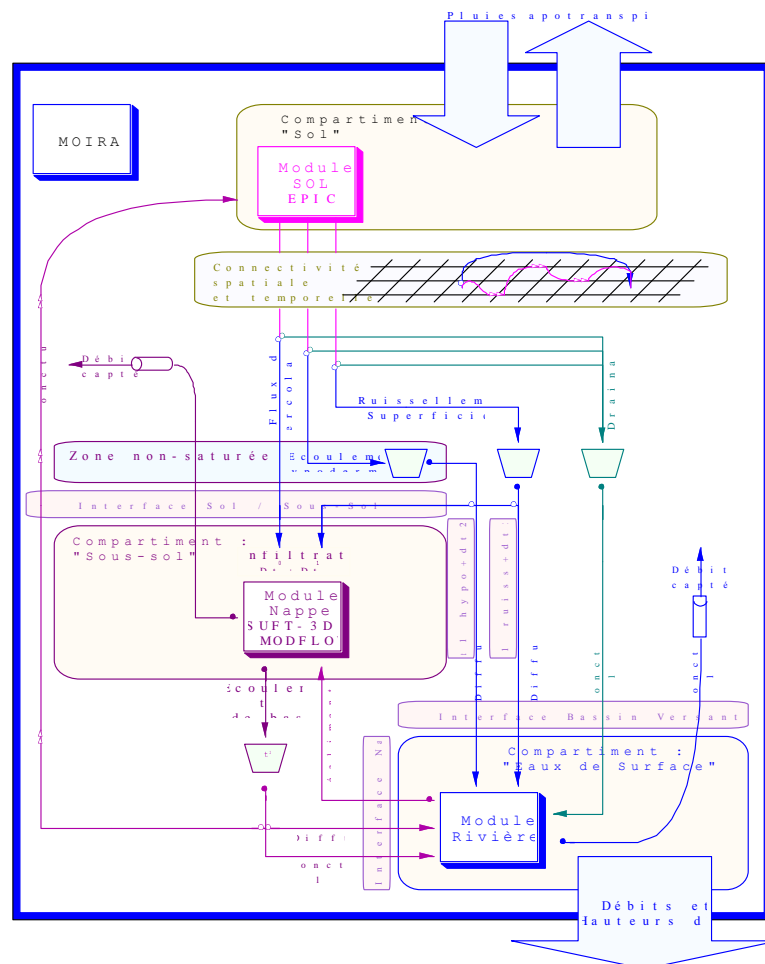
Figure 11 Architecture du modèle intégré MOIRA
