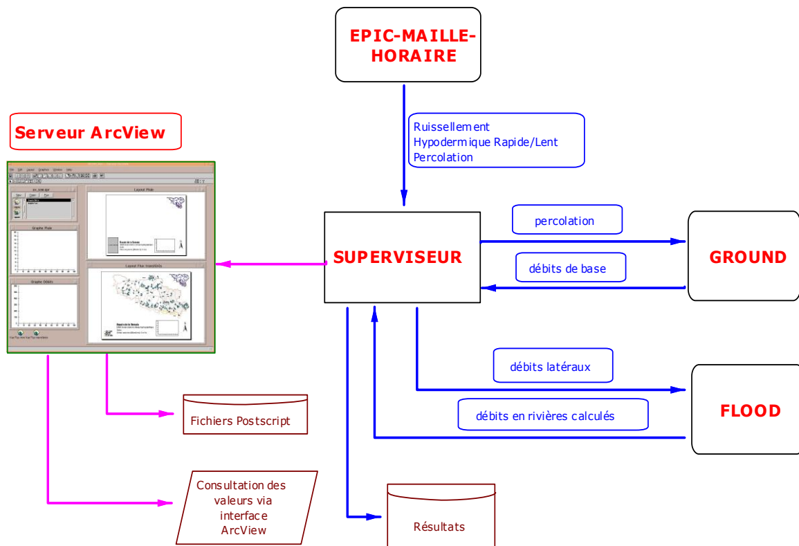
Figure 9 Architecture du modèle intégré MOHICAN
