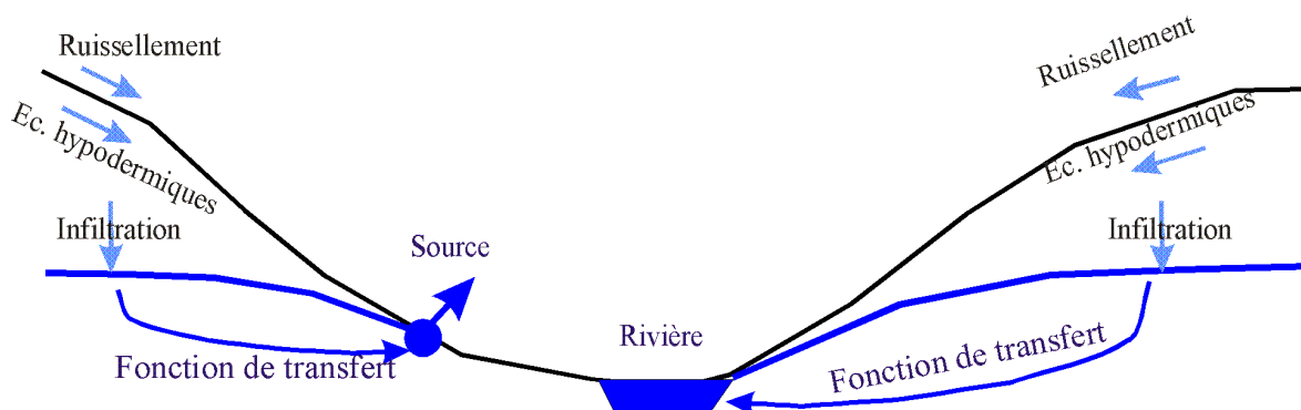
Figure 10 Schéma conceptuel des flux à l'échelle du bassin versant
