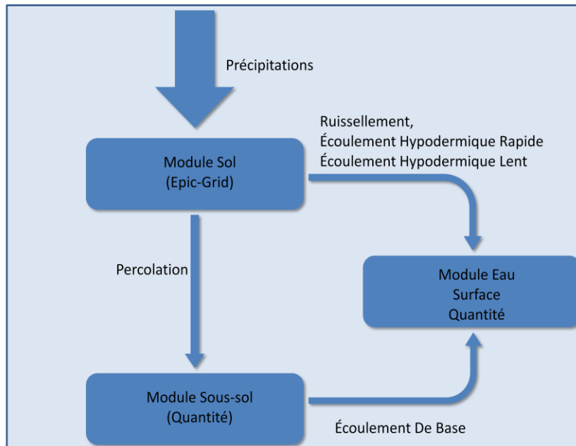
Figure 8 Architecture du modèle intégré MOHISE
