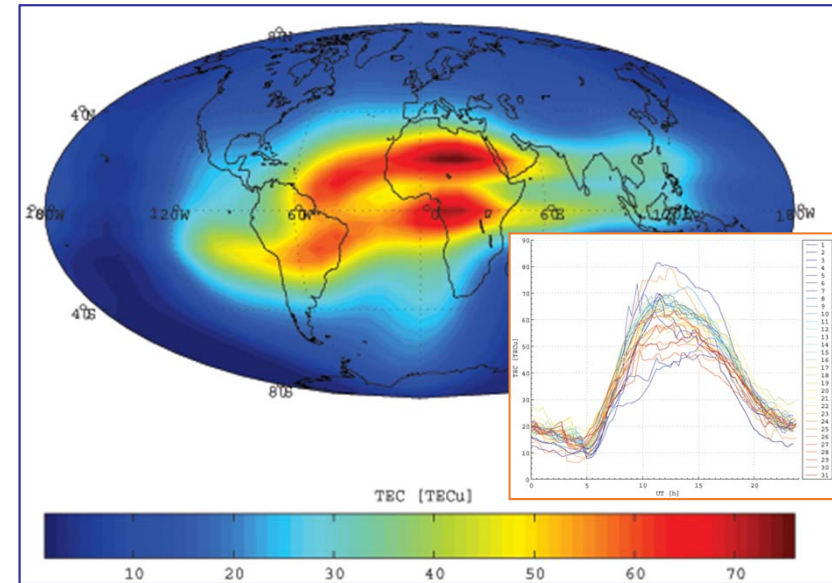
Contenu total en électrons et TEC journalier à Bruxelles
