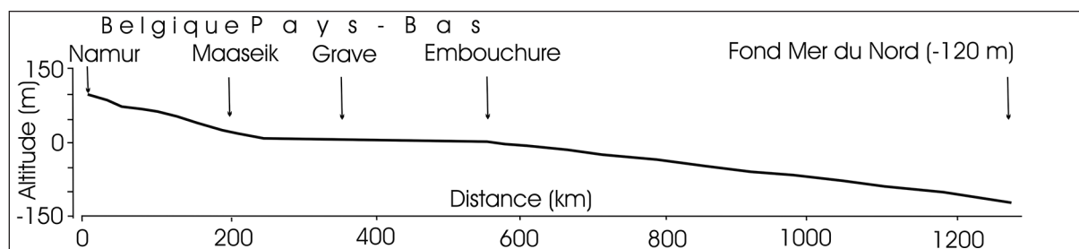
Figure 10. Pente longitudinale de la Meuse prolongée sur la plate-forme continentale de la Mer du Nord (exondée pendant les paroxysmes glaciaires).
