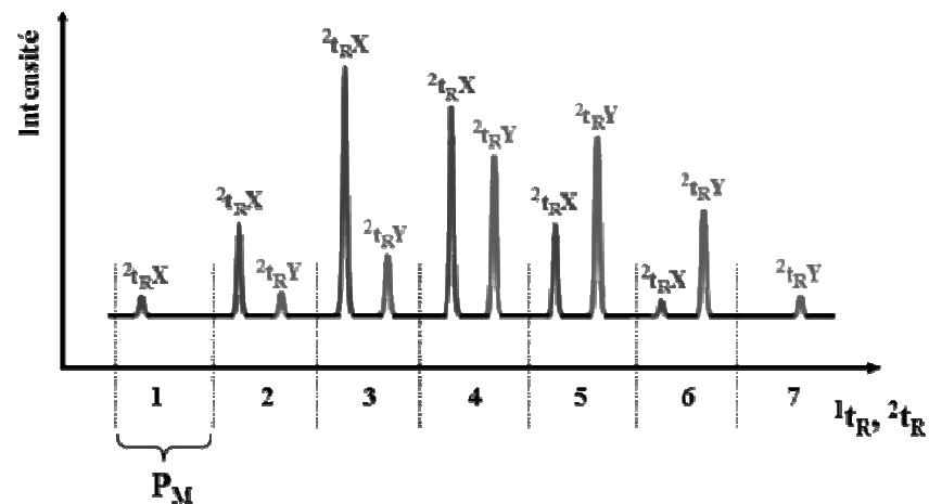
Figure 3 : Signal des données brutes enregistrées au détecteur (ref : J.-F. Focant, E. Reiner, K. MacPherson, J. Cochran, F. Dorman, A. Sjödin, D.G. Patterson Jr., Talanta 63 2004 1231-1240).
