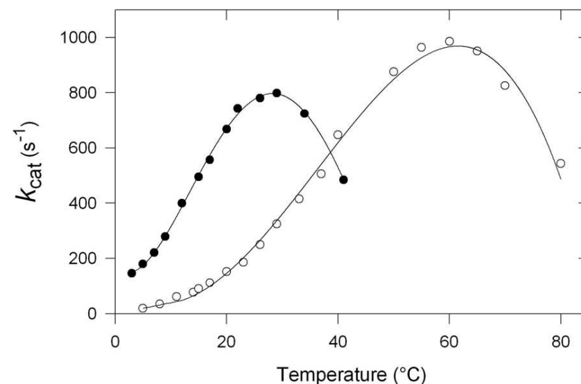
Figure 2. Activités spécifiques comparées en fonction de la température d'une \alpha -amylase psychrophile (points noirs), isolée d'une bactérie de l'antarctique Pseudoalteromonas haloplanktis , et d'une \alpha -amylase thermophile isolée de Bacillus amyloliquefaciens (points clairs).
