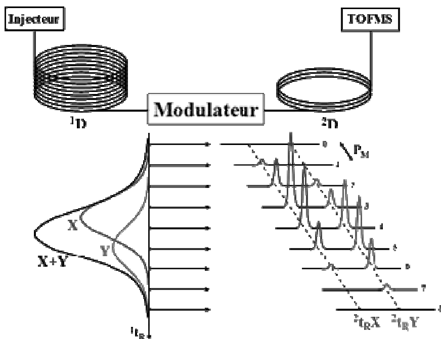
Figure 2 : Représentation schématique d'un modulateur en GCxGC (ref : J.-F. Focant, E. Reiner, K. MacPherson, J. Cochran, F. Dorman, A. Sjödin, D.G. Patterson Jr., Talanta 63 2004 1231-1240).
