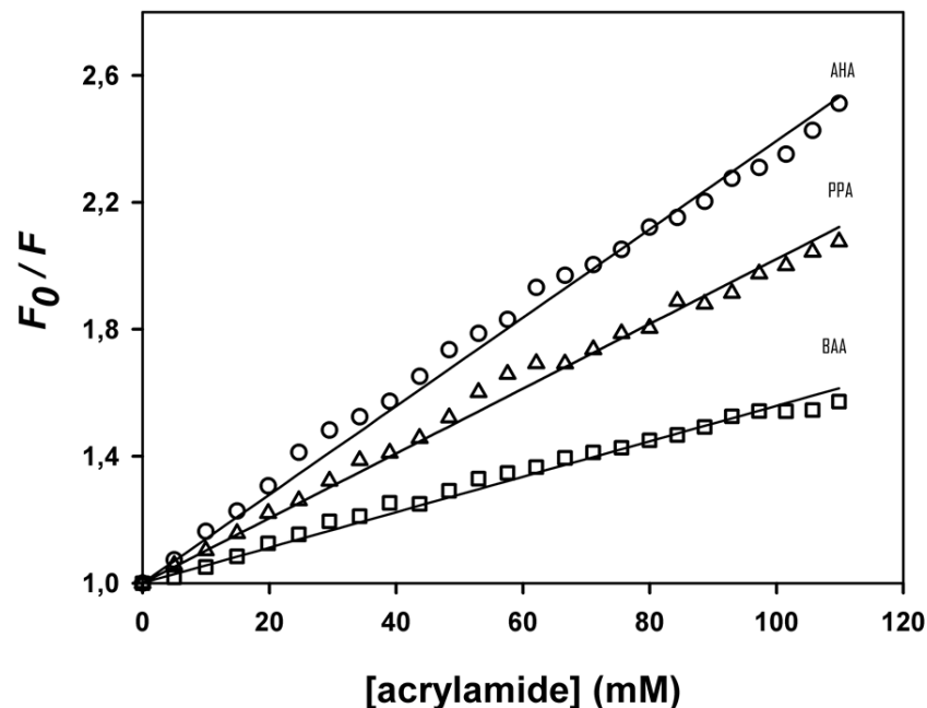
Figure 4. Quenching à l'acrylamide de la fluorescence d' \alpha -amylases psychrophile (AHA), mésophile (PPA) et thermophile (BAA). Le rapport F_0/F représente le rapport des fluorescences des enzymes avant et après l'ajout du quencher. Les pentes sont reliées à la facilité avec laquelle le « quencher » pénètre la structure tridimensionnelle.
