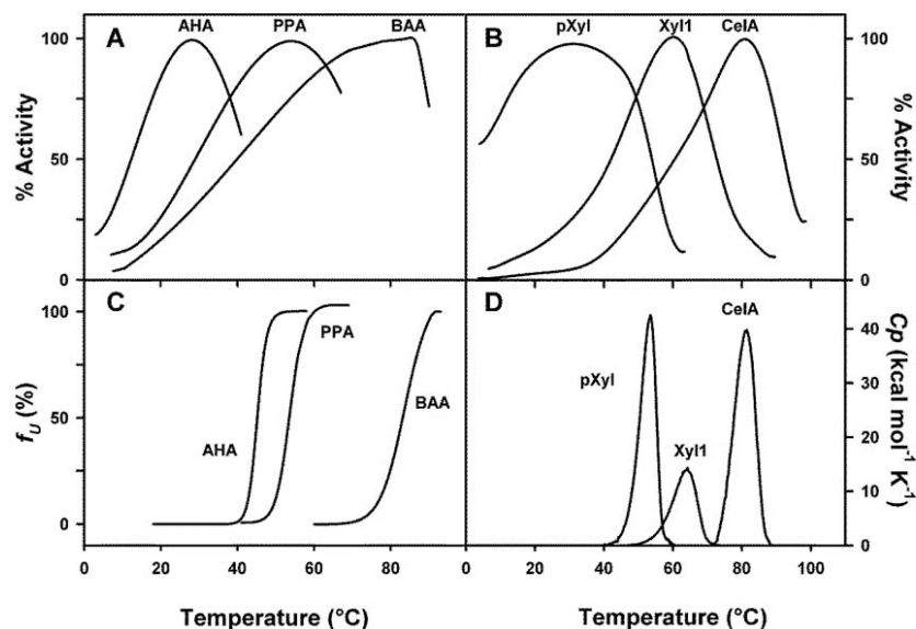
Figure 3. Inactivation (A) et stabilité thermique (C) d' \alpha -amylases psychrophiles (AHA), mésophile (PPA) et thermophile (BAA). Dans ce cas la dénaturation thermique est suivie par fluorescence. Inactivation (B) et stabilité thermique (D) d'une osidase psychrophile (pXyl), mésophile (Xyl1) et thermophile (CelA). Dans ce cas la dénaturation thermique est suivie par microcalorimétrie différentielle.
