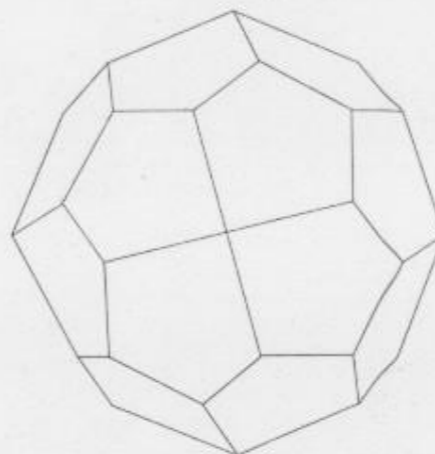
Épure XI' (Fig. 58)
