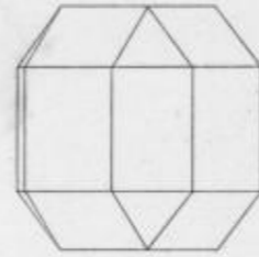
Épure VII (Fig. 39)
