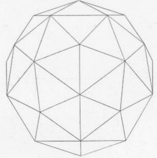
Épure V (Fig. 52)
