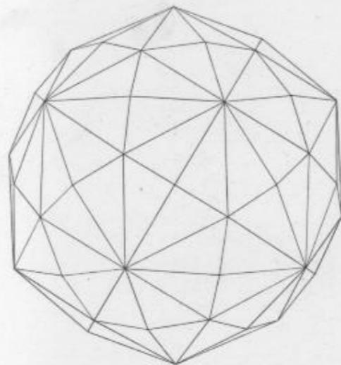
Épure XIV' (Fig. 63)
