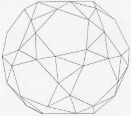
Épure XII (Fig. 49)
