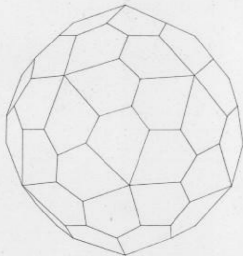
Épure XII' (Fig. 62)
