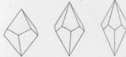
Épure VIII' (Fig. 42)
