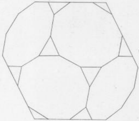
Épure III (Fig. 37.)
