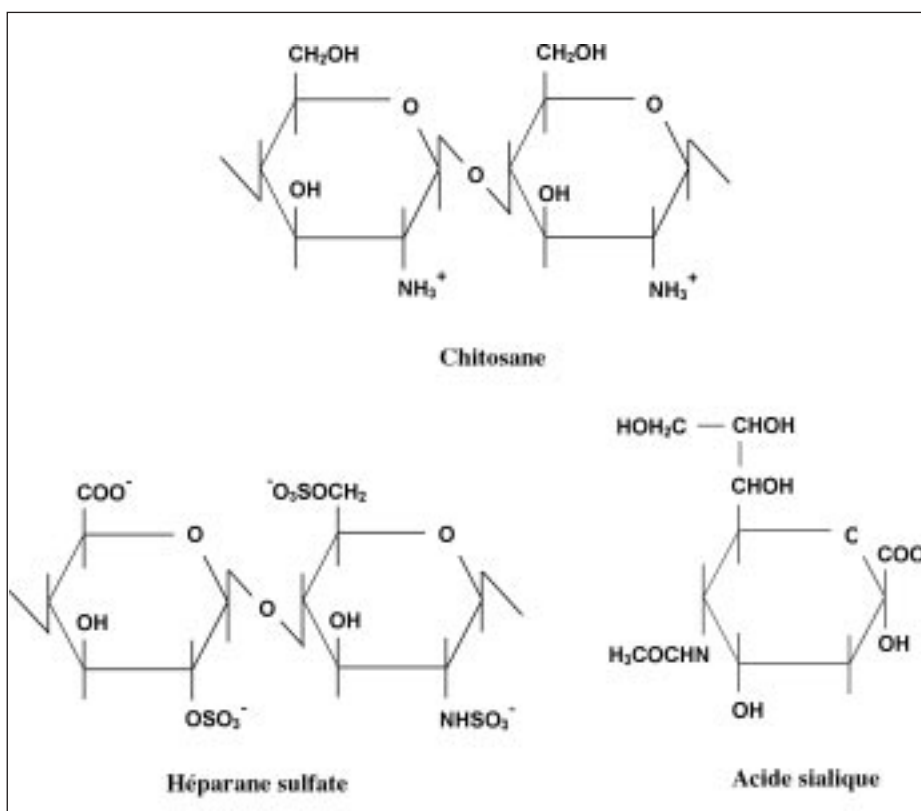
Figure 3: interactions chimiques formant des liaisons de type a) ionique entre les groupes amines ( -\text{NH}_3^+ ) chargés positivement du chitosane et le groupe carboxyle ( -\text{COO}^- ) de l'acide sialique et/ou les groupes carboxyles, ainsi que les groupes sulfates ( -\text{SO}_3^- ) d'héparane chargés négativement, et b) non ionique (les ponts d'hydrogène) entre les groupements hydroxyles ( -\text{CH}_2\text{OH} ) du chitosane, et les groupes carboxyles, hydroxyles et/ou sulfates des GAG en l'occurrence de l'héparane sulfate, ainsi que de l'acide sialique.
