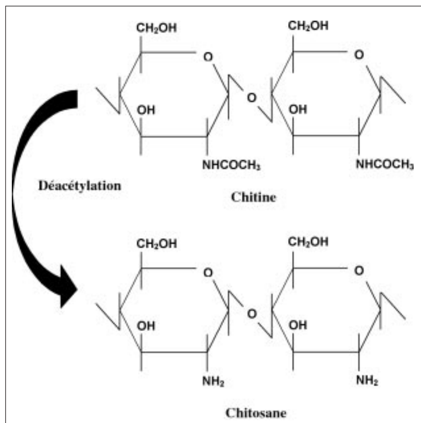
Figure 2: structures chimiques de la chitine et du chitosane. Ce dernier est obtenu par hydrolyse d'au moins 50% de groupes acétyle ( -CH_3CO ). Cette opération, appelée déacétylation, permet de libérer les groupes amines ( NH_2 ).
