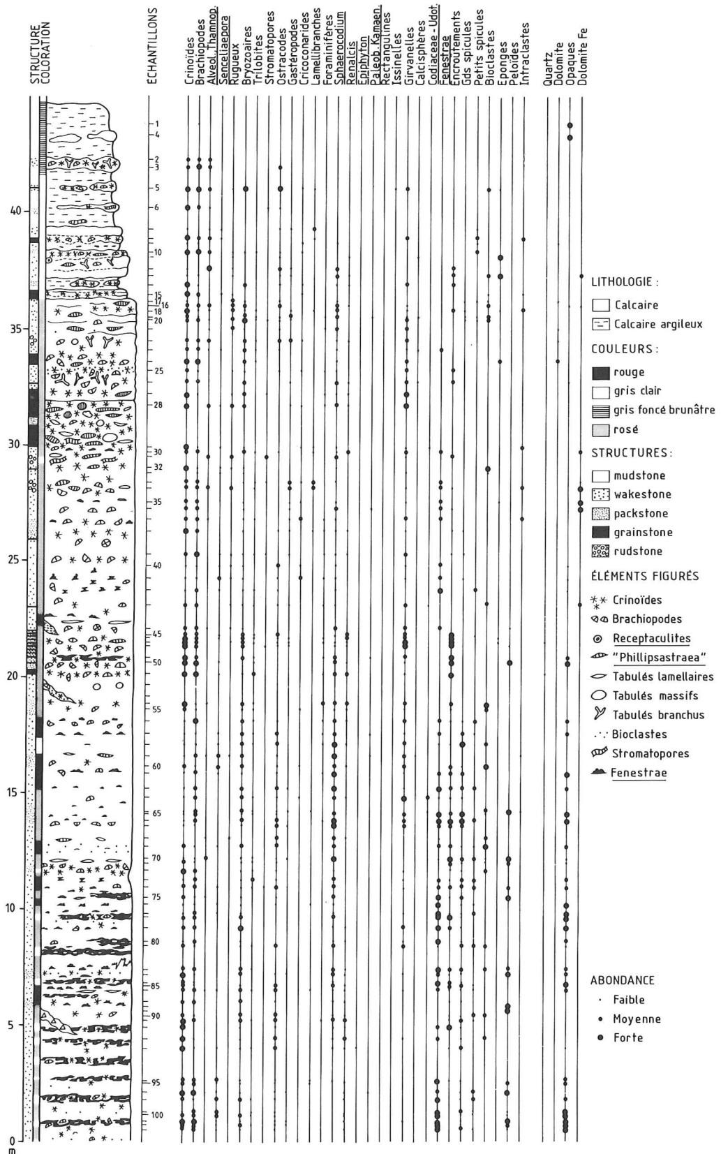
Figure 3.- Levé «banc par banc» de la paroi Est (coupe A de la fig. 2) de la carrière de Tapoumont et inventaire microscopique.
