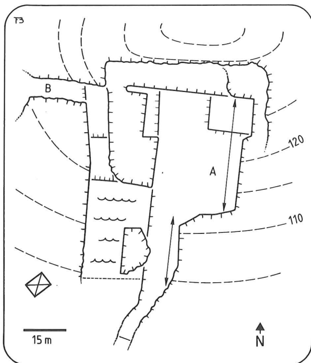
Figure 2 Plan de la carrière de Tapoumont au printemps 1987.
