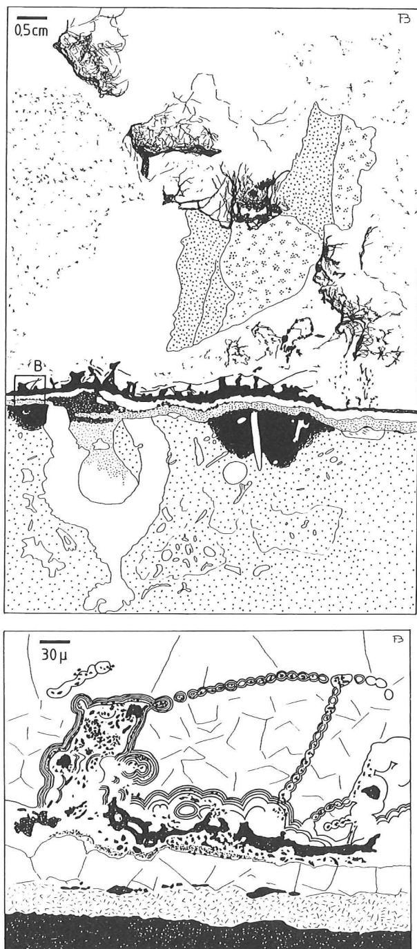
Figure 9.- lame mince ULB CR 1 (Vodecée, bloc scié). Remplissage de fissure, lumière transmise; la micrite est représentée par un pointillé, le ciment est blanc et les opaques sont noirs. Remarquer les nombreux filaments et les encroûtements complexes sur les parois. B. détail de A, lumière réfléchie, immersion d'huile; en noir, hématite, avec une structure concrétionnée, hydroxydes de fer.
