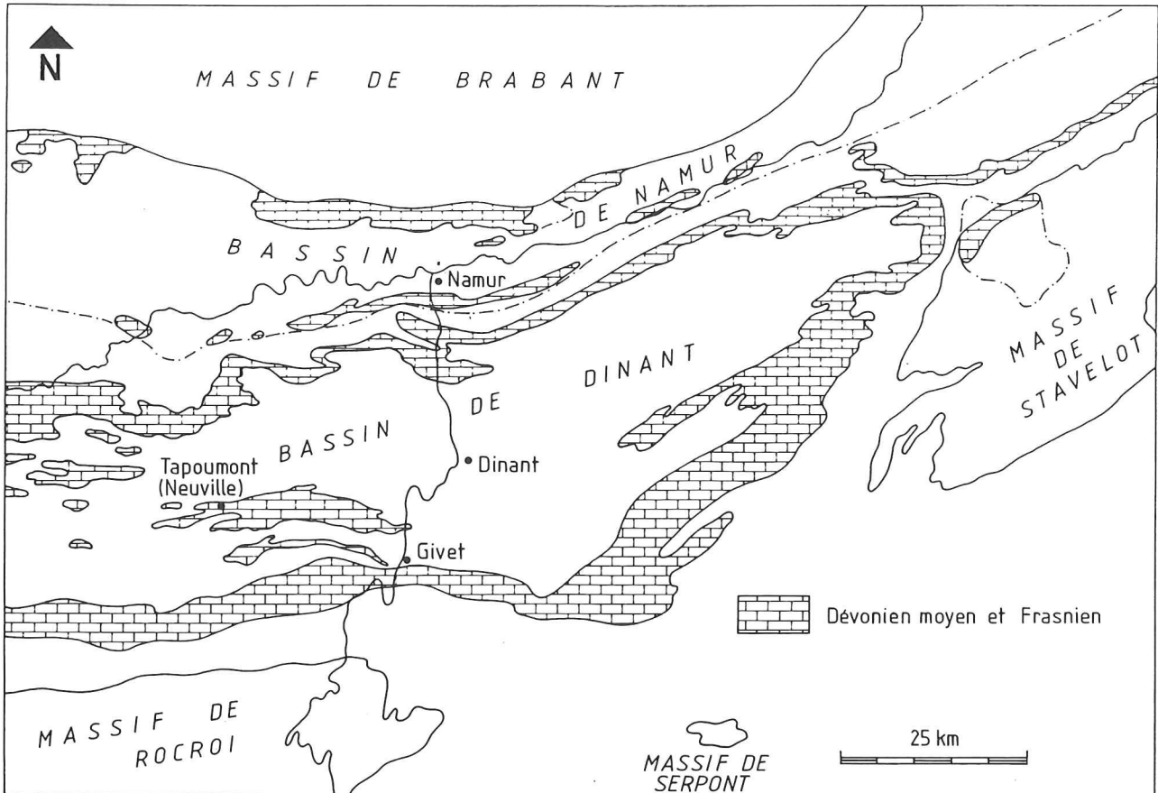
Figure 1 Carte géologique simplifiée du Sud de la Belgique; les coordonnées de la carrière de Tapoumont sont : 50° 09' 50" lat N et 4° 30' 16" long. E.
