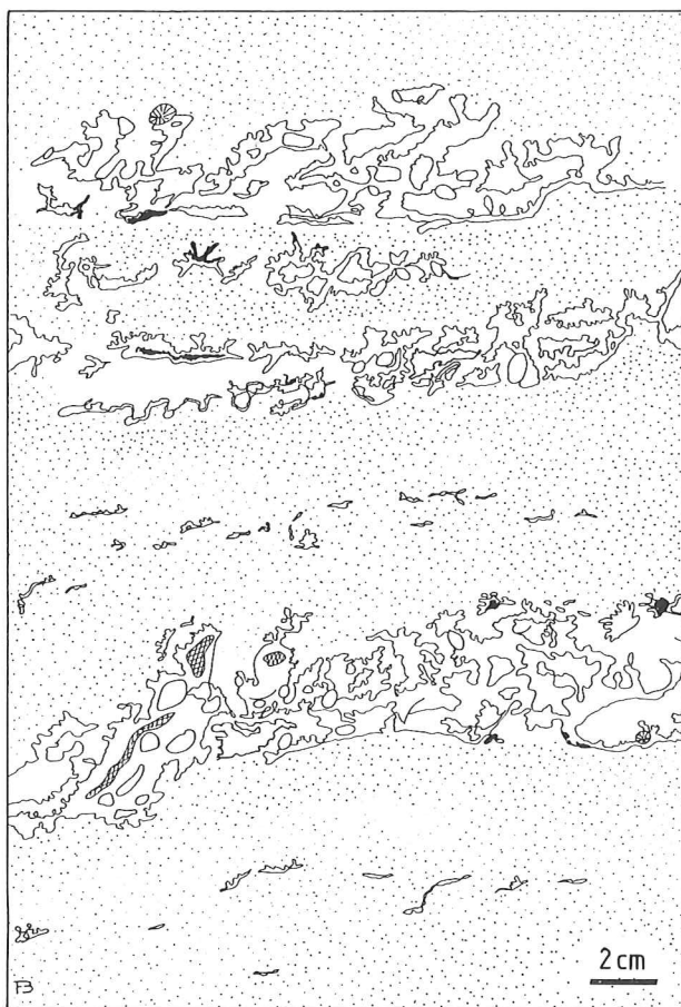
Figure 7.- Bloc scié, Tapoumont.
