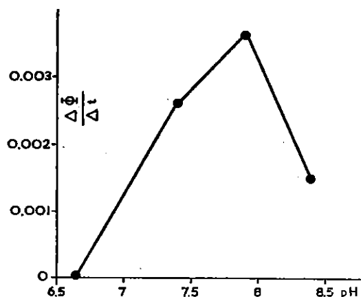
FIG. 13 Activité alginolytique, en fonction du pH, d'un extrait du tube digestif (courbure inférieure) de Psammochinus miliaris Gmelin.
