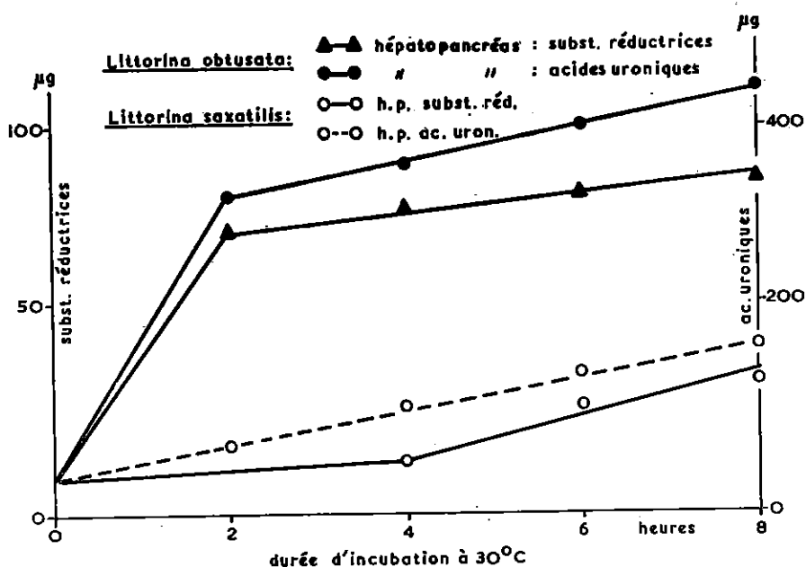
FIG. 6 Libération des sucres uroniques à partir d'alginate sous l'effet des extraits aqueux d'hépatopancréas de Littorina obtusata L. et de Littorina saxatilis L. (mesure des substances réductrices et des acides uroniques libérés, en µg de glucuronate/ml de milieu réactionnel).
