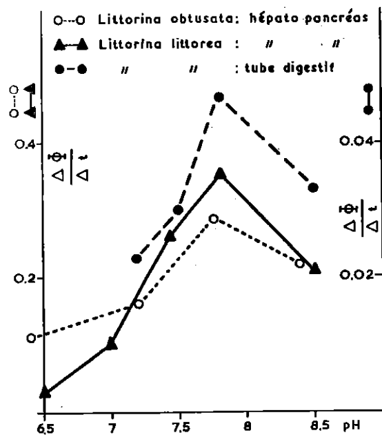
FIG. 4 Activité en fonction du pH, des extraits aqueux d'hépatopancréas de Littorina littorea L. et Littorina obtusata et du tube digestif de Littorina littorea .
