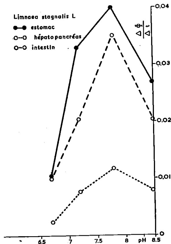
FIG. 10 Activité alginolytique en fonction du pH, des ex- traits d'hépatopancréas d'intestin et d'estomac de Limnaea stagnalis L.
