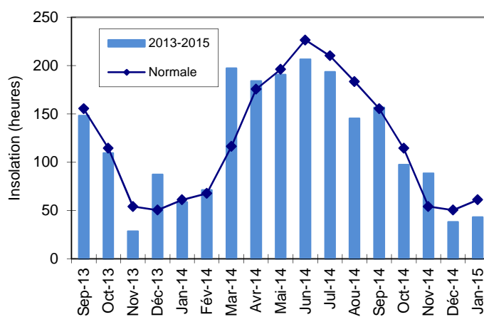
Figure 1.11 – Insolation mensuelles de septembre 2013 à janvier 2015 au poste climatologique d'Ernage-Gembloux (CRA-W).
