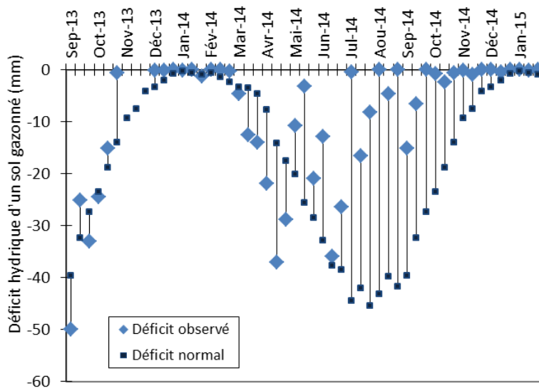
Figure 1.15 – Evolution du déficit hydrique d'un sol gazonné de septembre 2013 à janvier 2015.
