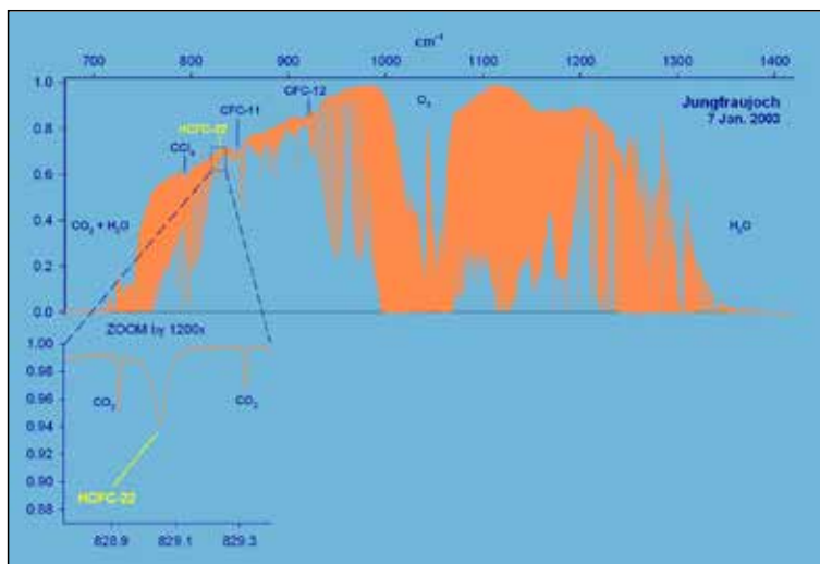
Figure 4 : Spectre FTIR typique entre 7 et 14 micromètres. Des absorptions par l'ozone, la vapeur d'eau, le dioxyde de carbone (CO 2 ) y sont identifiées. La partie inférieure montre une portion du spectre agrandie 1200 fois, permettant de visualiser une signature spectrale associée au HCFC-22.
