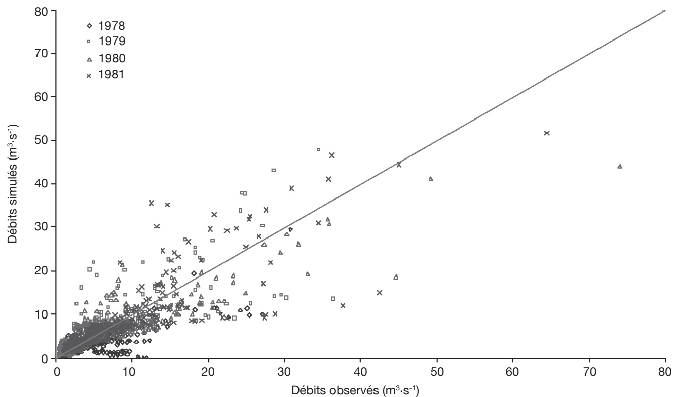
Figure 2. Ourthe à Mabompré (319 km 2 ) : comparaison des débits journaliers observés et simulés, calage automatique : années 1978-1981 — Ourthe in Mabompré (319 km 2 ): observed and simulated daily flows, self-calibration: years 1978-1981.
