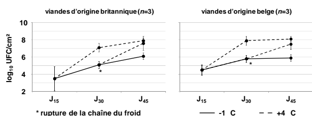
Figure 1 Dénombrement de la flore aérobie totale ( +22^{\circ}\text{C} ) dans des échantillons de viande fraîche. Les courbes représentent la tendance de croissance
