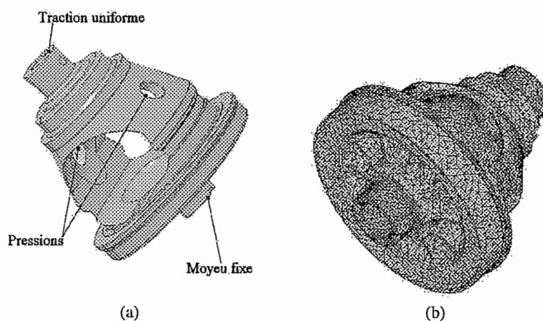
Figure 5. Modèle simplifié de l'étude d'un carter de différentiel (Renault).
