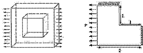
Figure 3. Pièce trouée soumise à traction uni-axiale.
