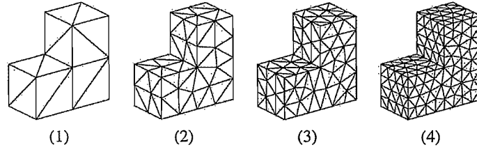
Figure 4. Maillages de la pièce trouée.
