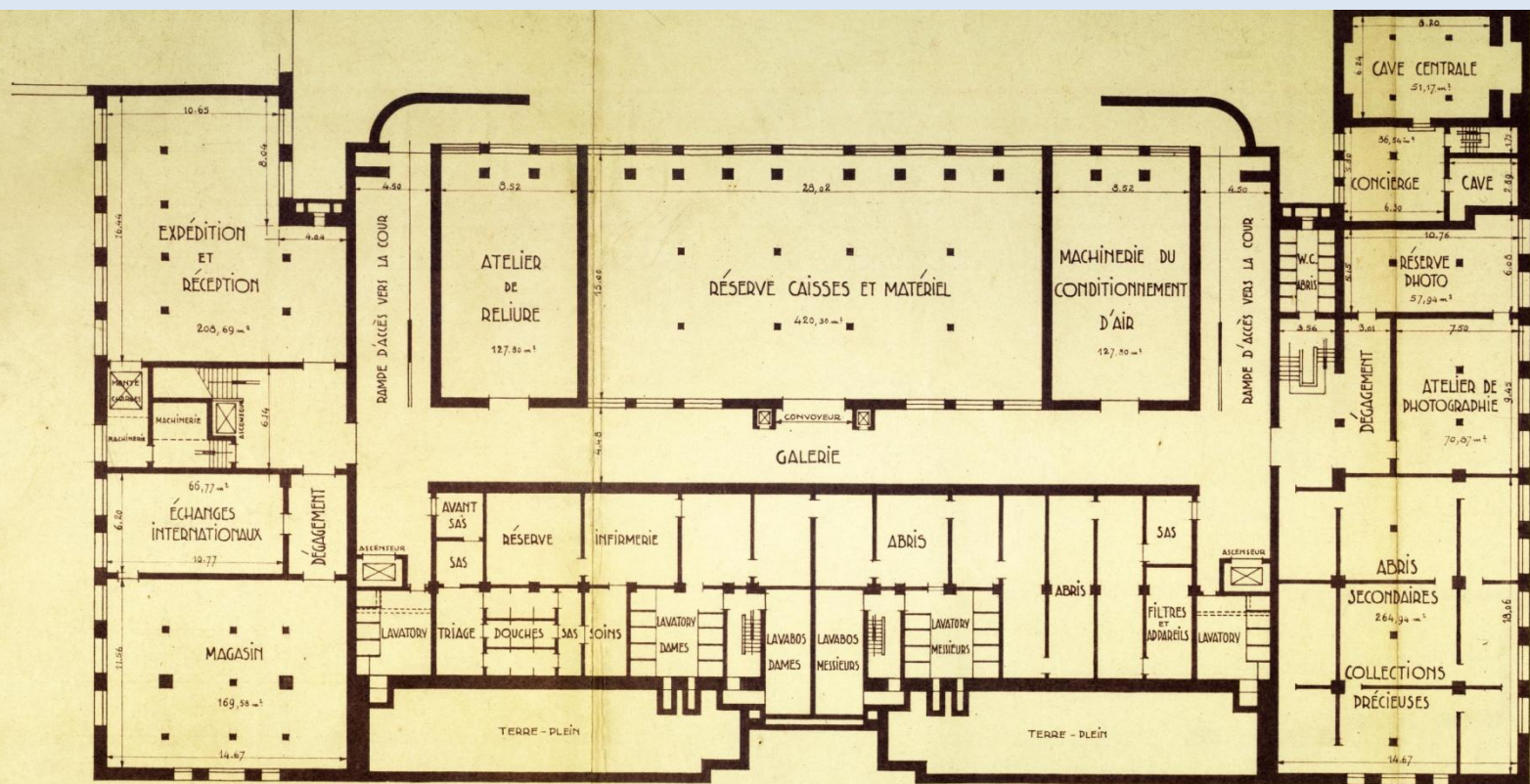
PLAN DU SOUS-SOL
