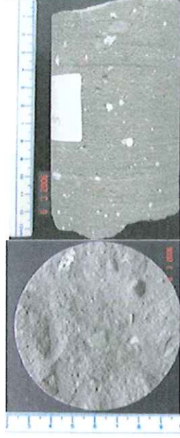
Figura 1. Testemunho de furo raso da Themag, cortado em diamictitos da Formação Poti na região de Itapititins (TO), apresentando clastos de natureza diversa.
