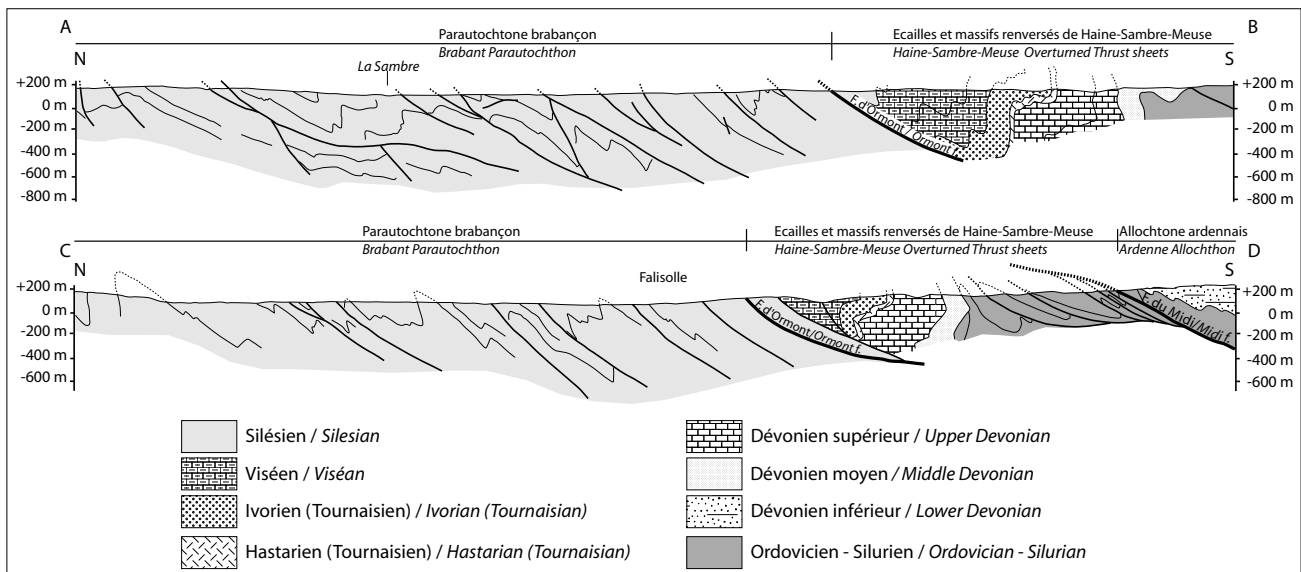
Fig. 3 : Coupes méridiennes sur la carte Tames – Fosses-la-Ville (Delcambre et Pingot, sous presse a). AB et CD se réfèrent aux lignes de coupe situées à la Fig. 5. NS cross sections of Tames – Fosses-la-Ville (Delcambre & Pingot, sous presse a). AB and CD refer to cross section lines of Fig. 5.
