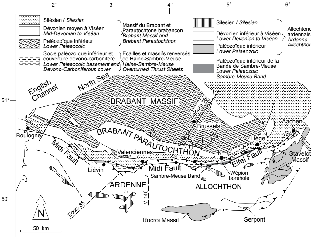
Fig. 1 : Le front varisque dans son contexte lithostratigraphique en Belgique et dans les pays limitrophes ; localisation des grands profils sismiques (tiré de Hance et al. , 1999). Abbreviations : B : Binche ; C : Charleroi ; H : Huy ; N : Namur. Lithostratigraphic context of the Variscan Front in Belgium and adjacent countries ; situations of major seismic profiles (from Hance et al. , 1999). Abbreviations : B : Binche ; C : Charleroi ; H : Huy ; N : Namur.
