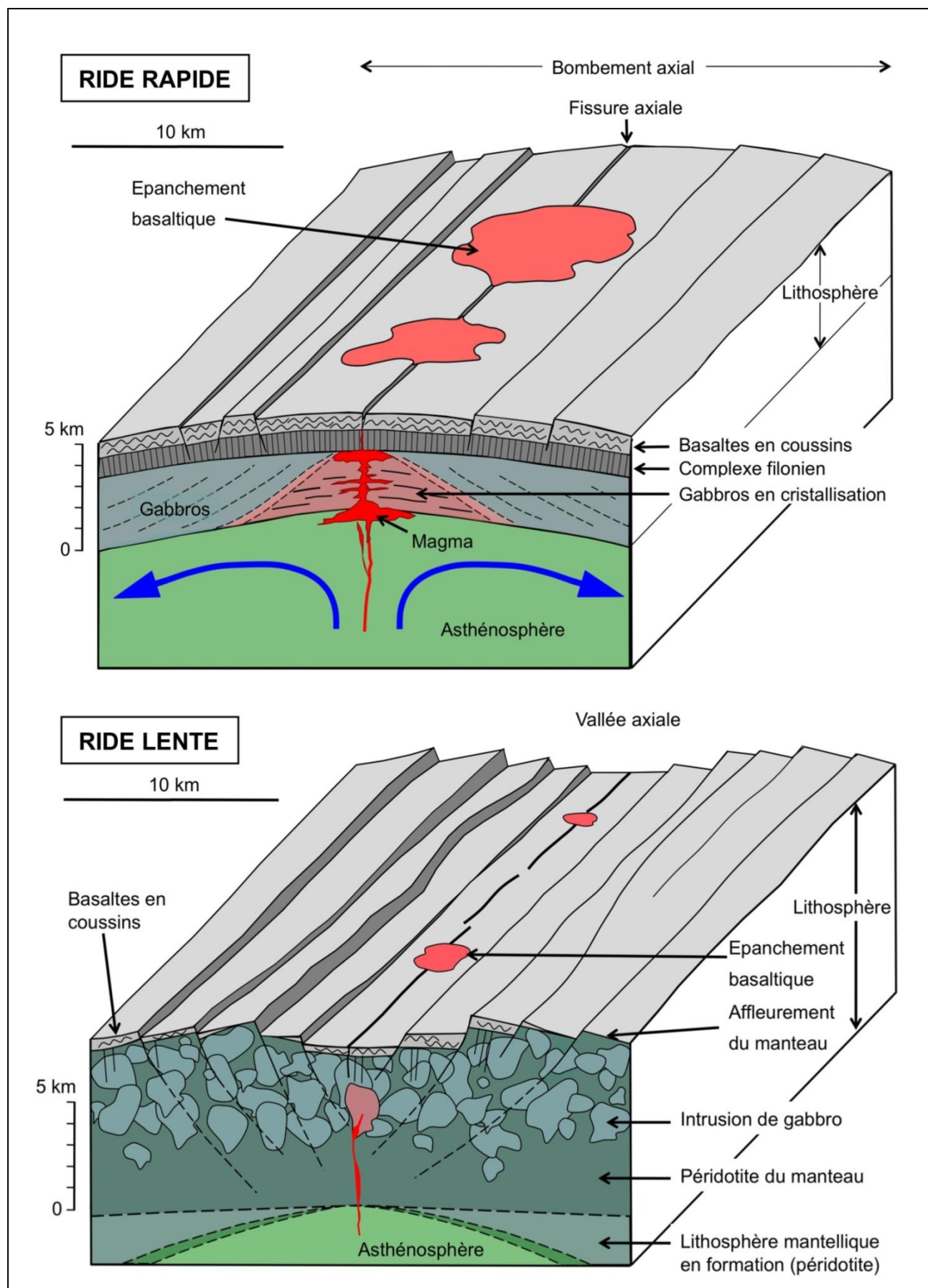
Géomorphologie et coupes géologiques dans une ride « rapide » (en haut) et dans une ride « lente » (en bas).
