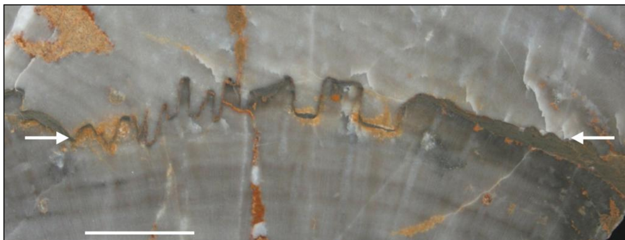
Stylolithe développé au contact de deux colonies calcaires de coraux fossiles (entre les deux flèches). La longueur du trait est de 2 cm.
