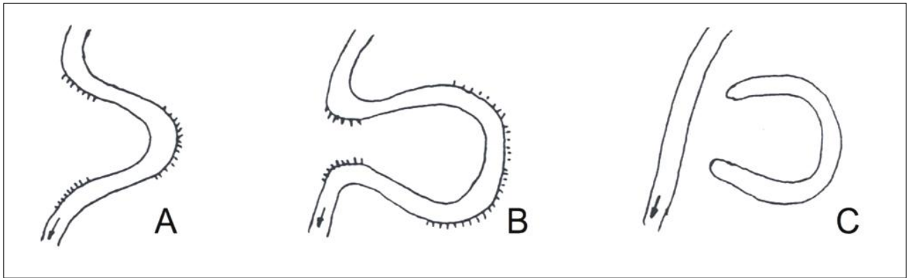
Schéma de formation d'un méandre recoupé.
