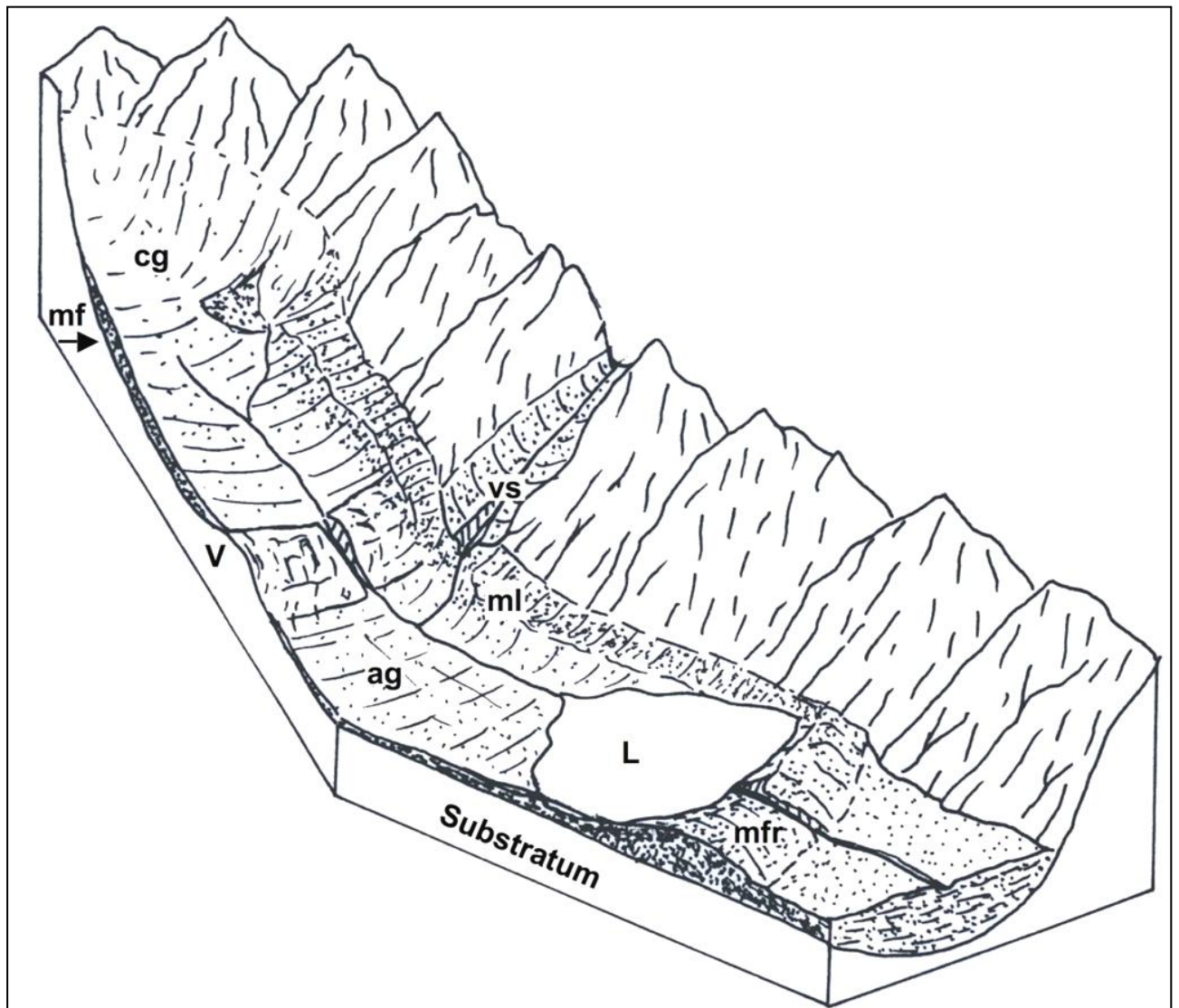
Relief glaciaire. ag, auge glaciaire ; cg, cirque glaciaire ; L, lac de barrage ; mf, moraine de fond ; mfr, moraine frontale ; ml, moraine latérale ; V, verrou glaciaire ; vs, vallée glaciaire suspendue.
