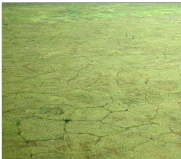
A gauche, sols polygonaux périglaciaires ; à droite, pingo dans la taïga. Omolon, NE Sibérie.
