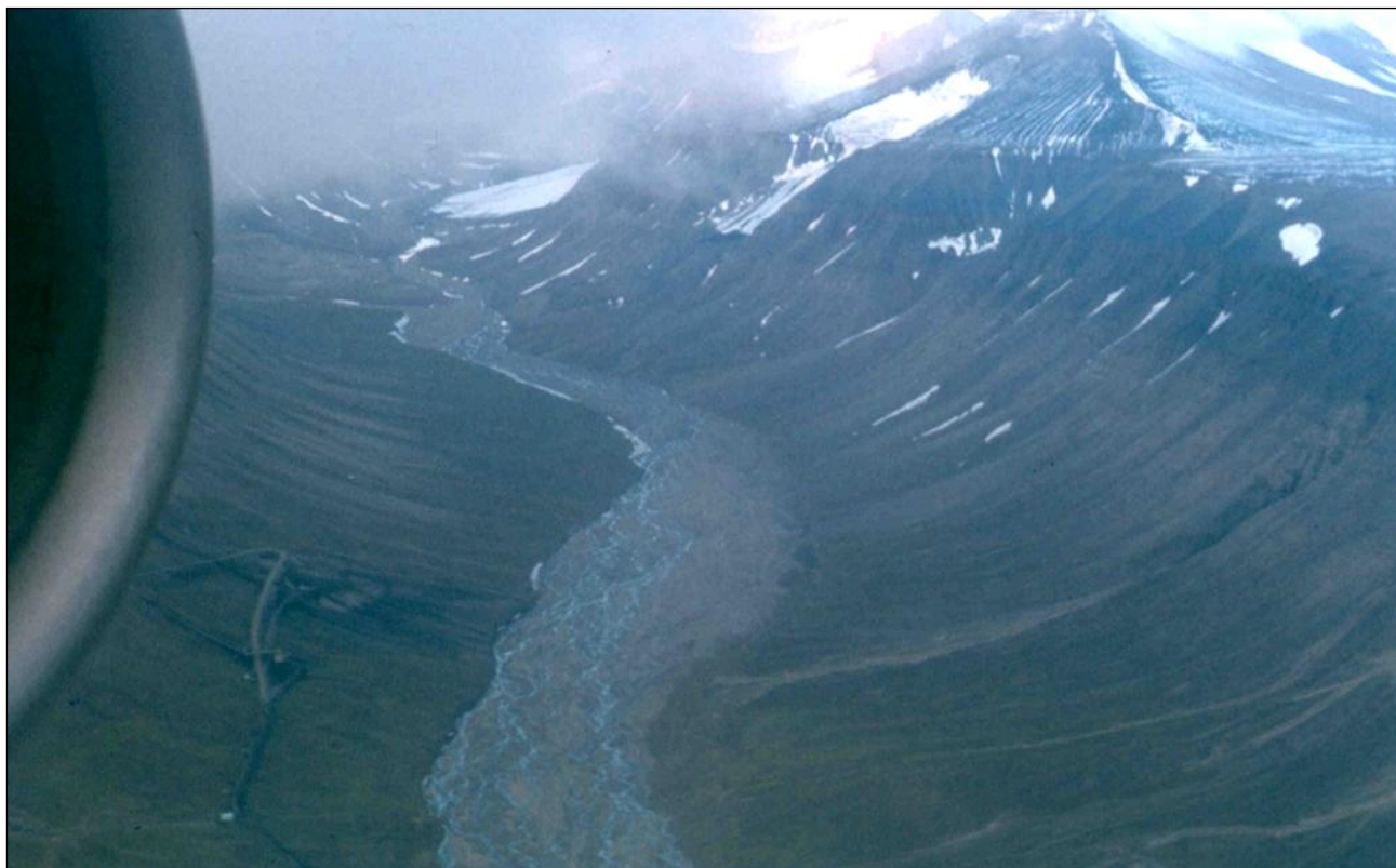
Vallée glaciaire en auge au Spitsberg.
