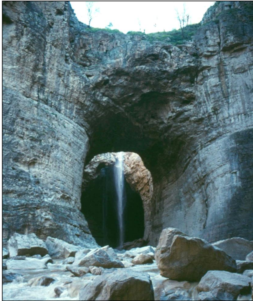
Conduit karstique évoluant en gorge suite à l'effondrement progressif de sa voûte (Gorge du Rummel, Constantine, Algérie).
