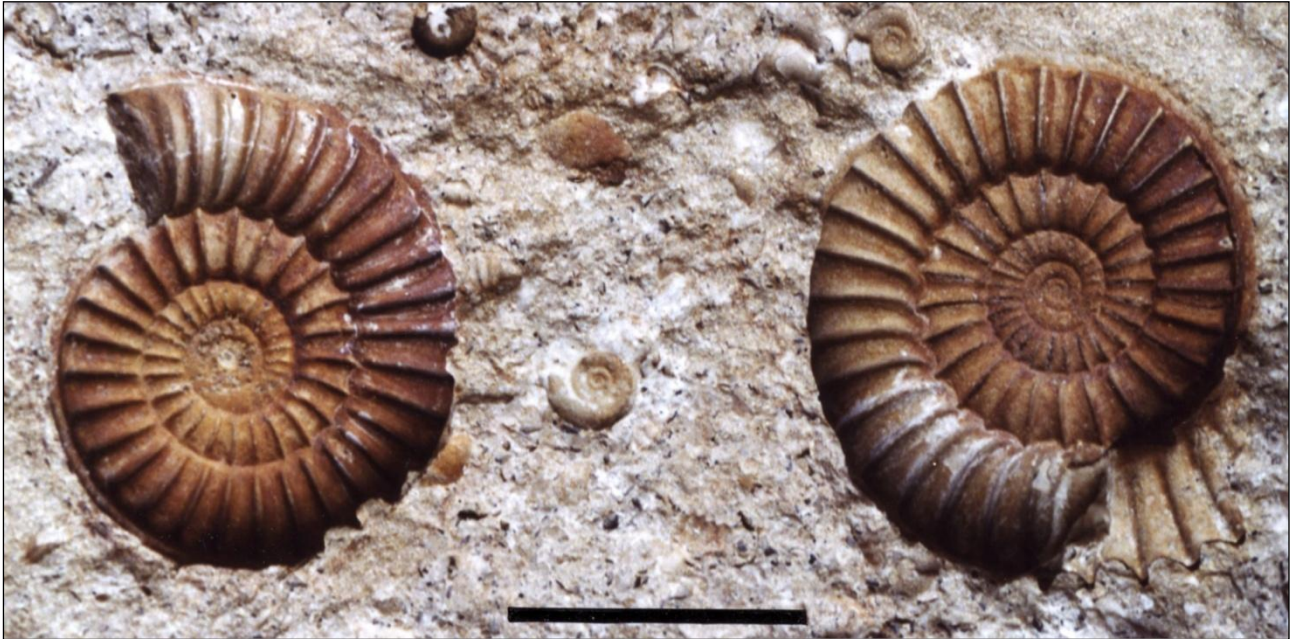
Ammonites du Jurassique inférieur du sud de la Belgique (Gaume). Le trait vaut 5 cm.
