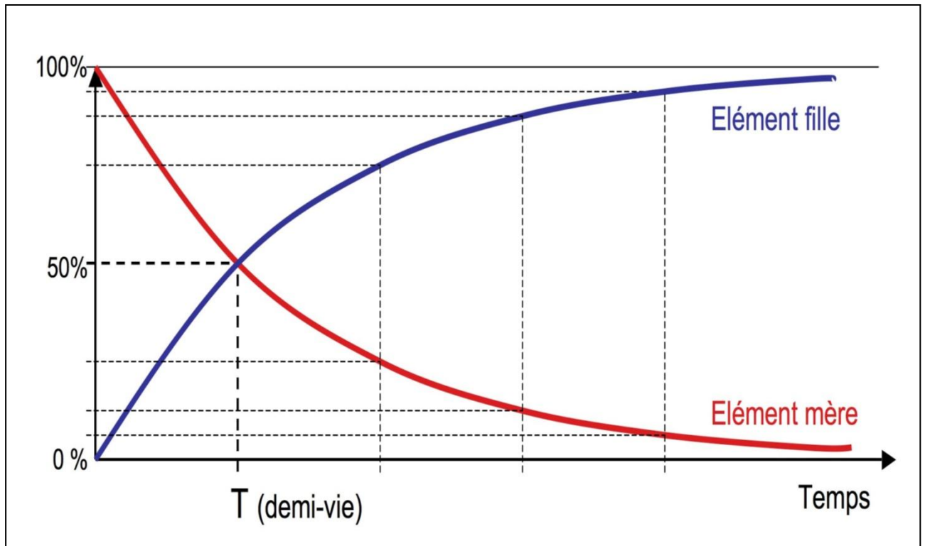
Diagramme de modification d'un élément radiogénique en fonction du temps.
