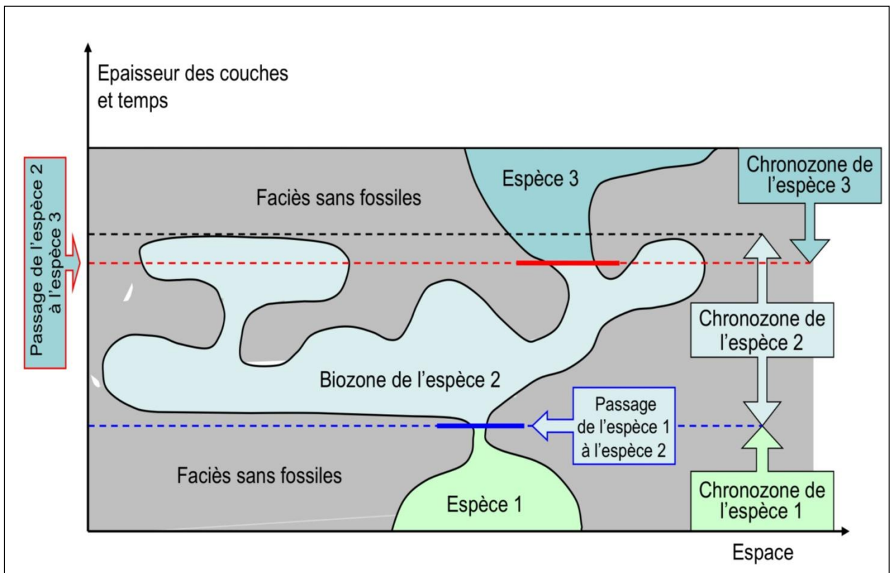
Répartition spatio-temporelle (biozone) de trois espèces liées phylétiquement. Dans le schéma, l'espèce 2 donne naissance à l'espèce 3 avant son extinction. La chronozone de l'espèce 3 couvre par conséquent en partie celle de l'espèce 2.
