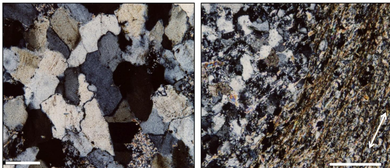
A gauche, quartzite diagénétique du Famennien ; à droite, quartzophyllade de l'Ordovicien du Massif de Stavelot (microquartzite à gauche de la photo, fins minéraux micacés à droite). Le trait vaut 2 mm, la double flèche indique le plan de schistosité.
