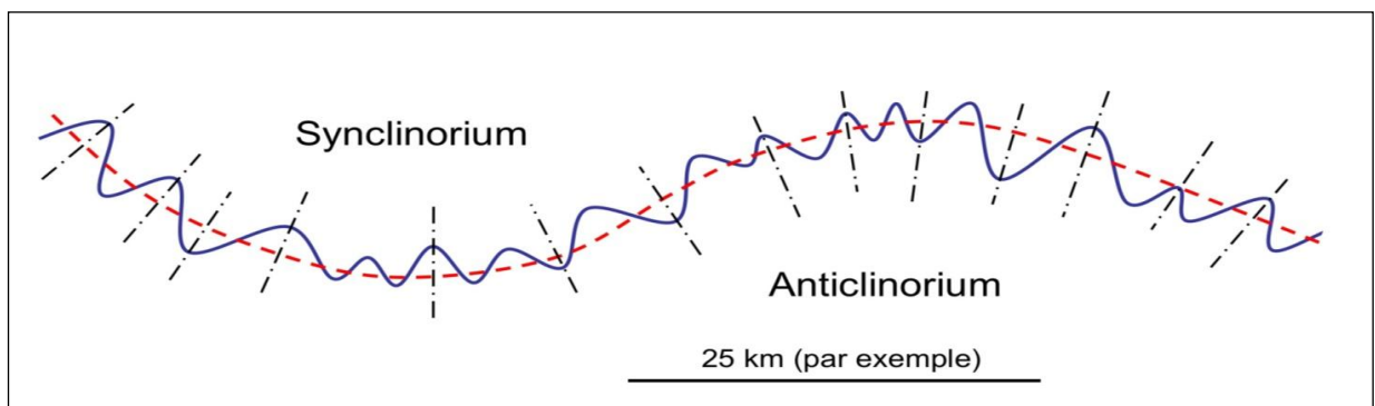
Synclinorium et anticlinorium.
