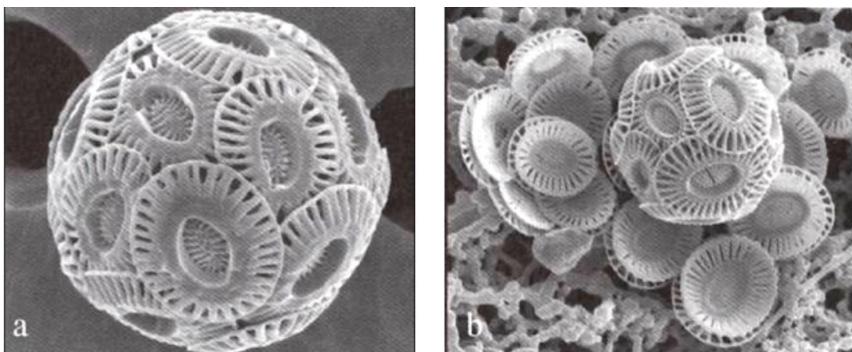
a : Coccolithophoridé actuel (environ 10 \mu\text{m} de diamètre); b : coccolithophoridé dissociés en coccolithes. La frustule est composée de plusieurs couches concentriques de coccolithes.
