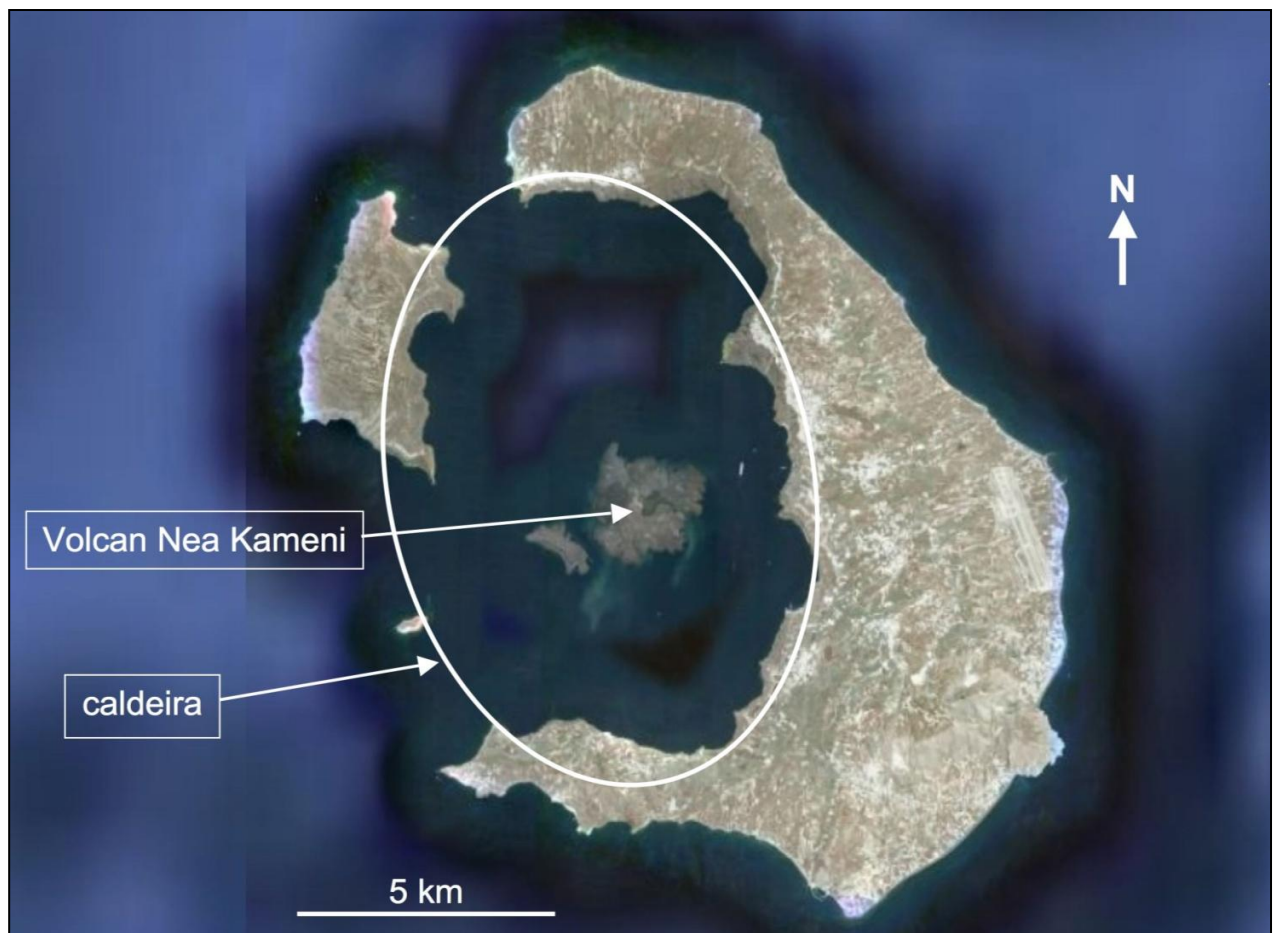
Vue aérienne de l'archipel de Santorin dans la mer Egée et de sa caldeira. Un nouvel édifice volcanique, Nea Kameni, dont la dernière éruption remonte à 1950, s'est progressivement développé au centre de la caldeira.
