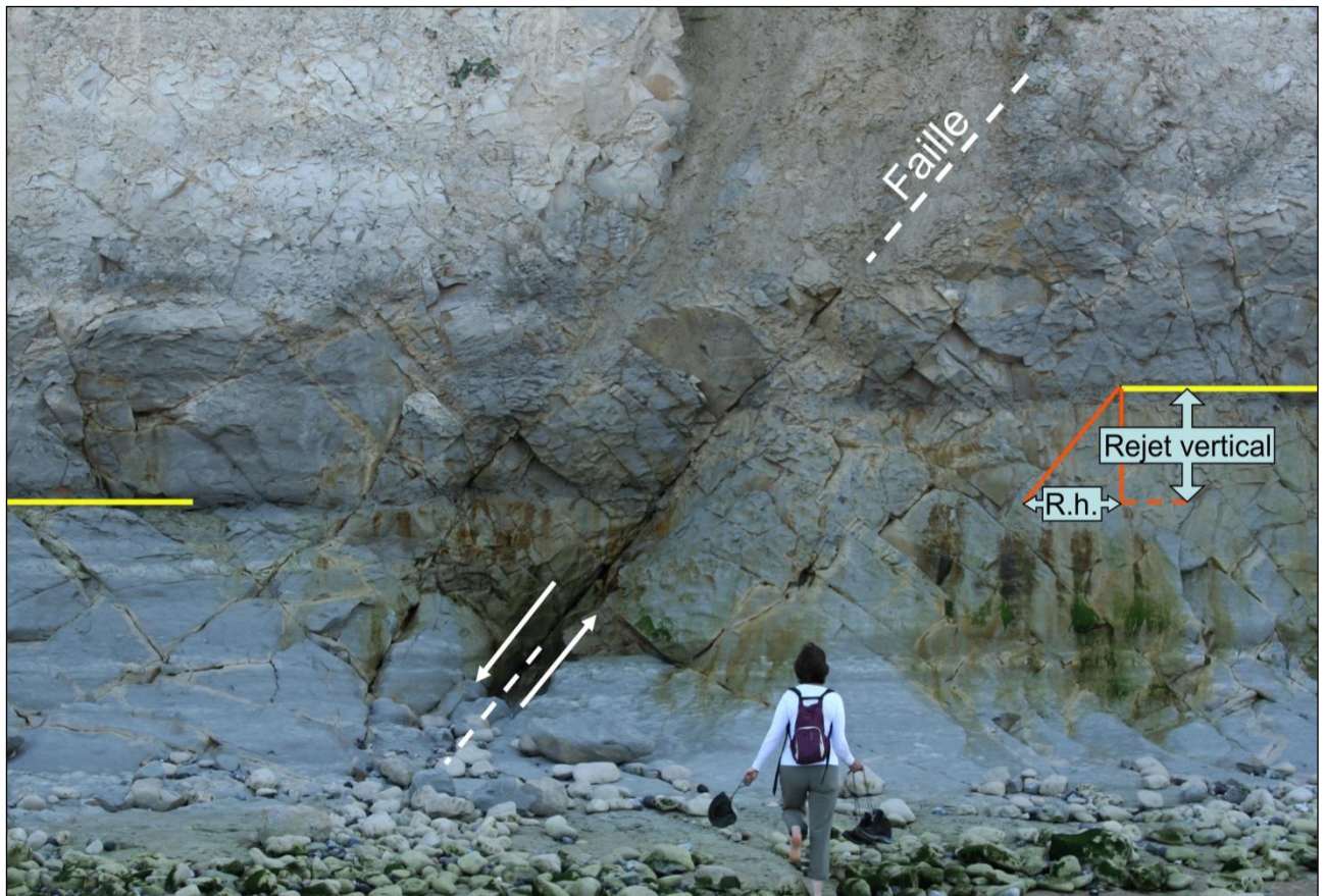
Faille normale dans la craie du Crétacé supérieur du Boulonnais. Les traits jaunes marquent un niveau repère qui permet de visualiser le rejet de la faille (indiqué et décomposé à droite ; R.h. = rejet horizontal).
