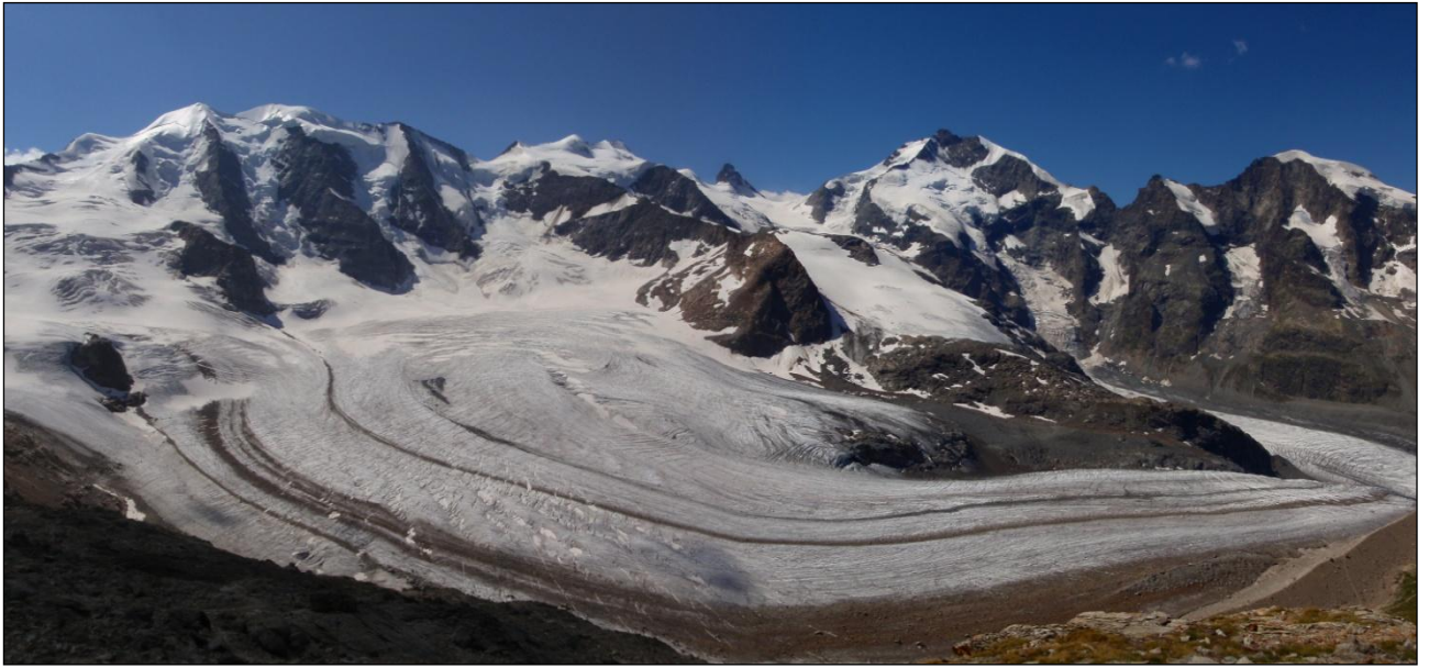
Moraines médianes. Glacier Pers, Massif de la Bernina, Suisse .
