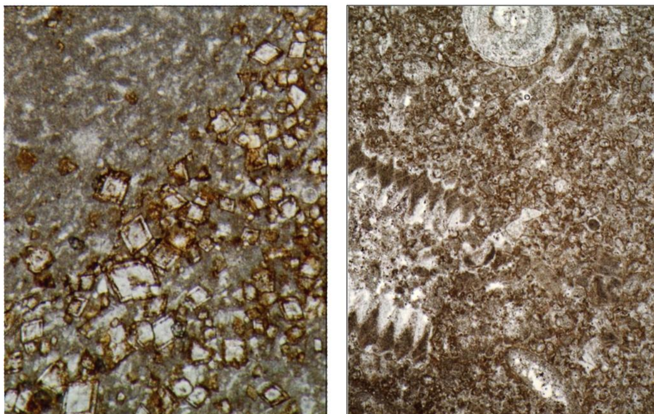
A gauche, cristaux de dolomite dans un calcaire partiellement dolomitisé ; à droite, dolomie renfermant des « fantômes » d'articles de crinoïdes qui montrent que la roche d'origine était un calcaire à crinoïdes.
