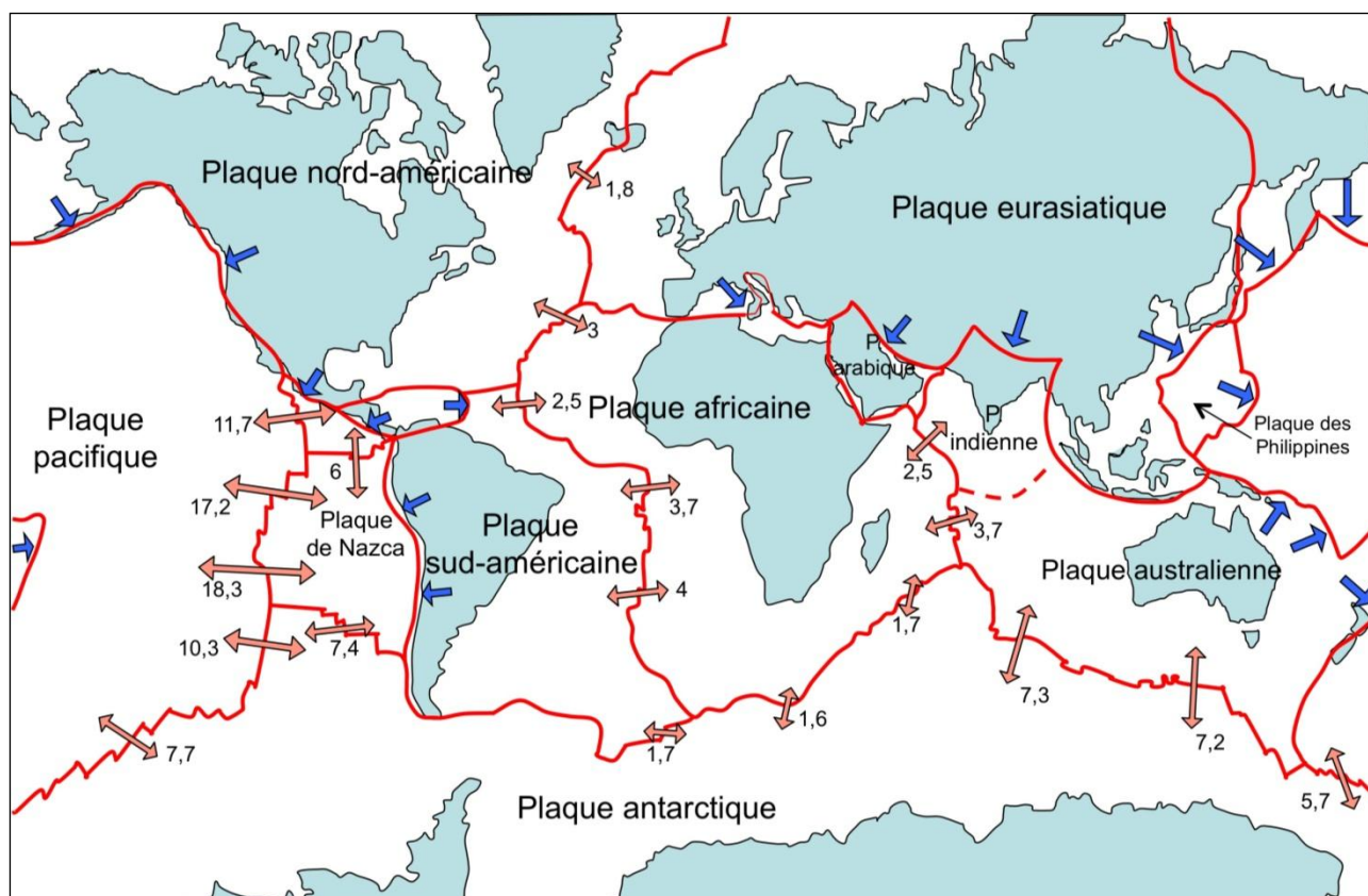
Principales plaques lithosphériques et variation des vitesses relatives d'expansion des plaques à l'endroit des dorsales en cm/an. Doubles flèches : zones d'accrétion ; flèches bleues : zones de convergence.
